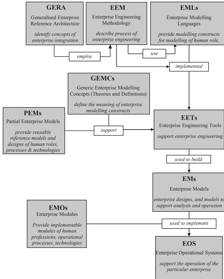
figure II.13 : Eléments méthodologiques de GERAM [IFIP 99]
