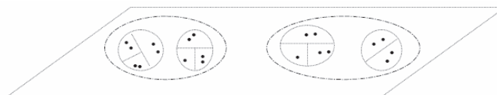
figure V.49 : Méthode de classification hiérarchique descendante
