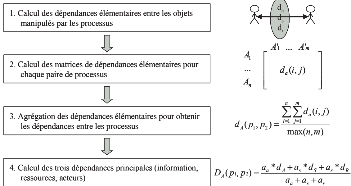
figure V.46 : Représentation schématique du mécanisme d'agrégation pour la dépendance d'acteur
