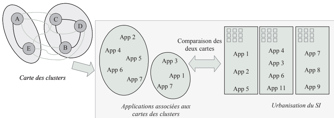
figure VI.60 : Principe de comparaison entre les clusters issus de la carte générale et les clusters de l'urbanisme du système informatique
