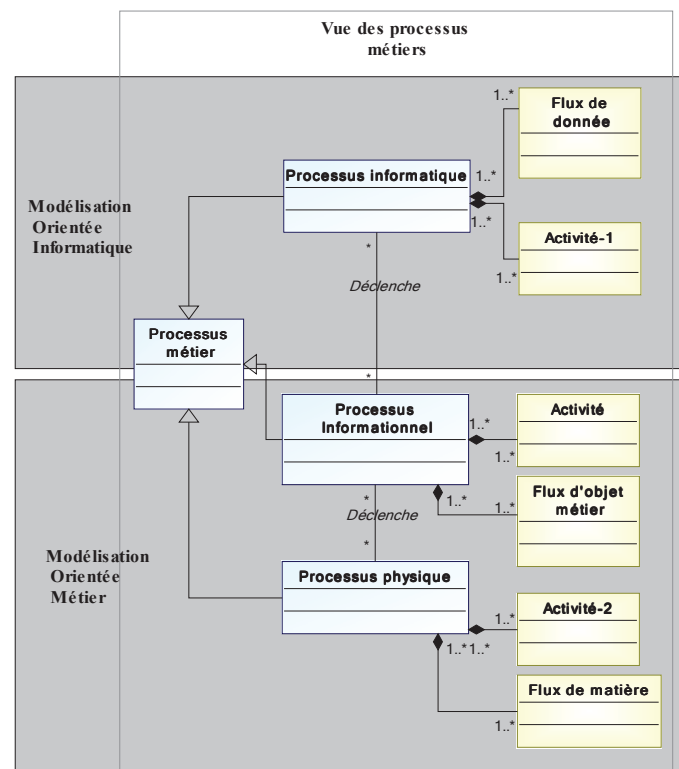
figure IV.33 : Vue des processus métiers
