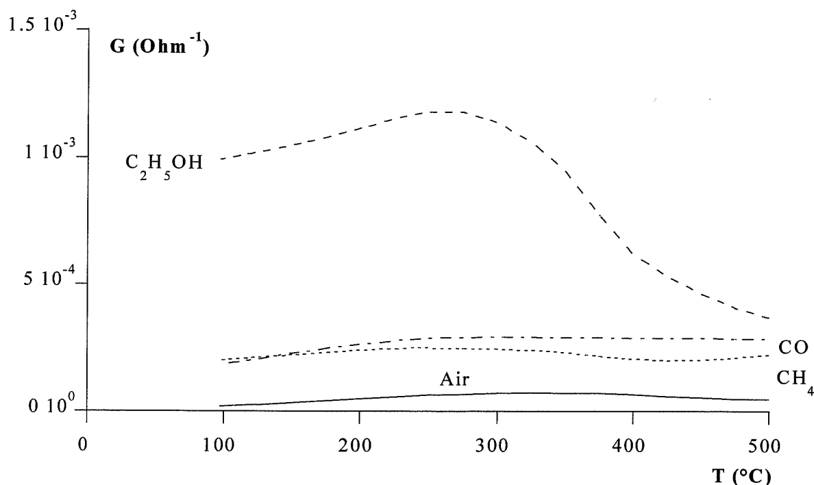
Figure II.13. courbes G = f(T) pour une couche obtenue par évaporation. Air ; C_2H_5OH = 100 ppm dans l'air ; CO = 300 ppm dans l'air ; CH_4 = 1000 ppm dans l'air.
