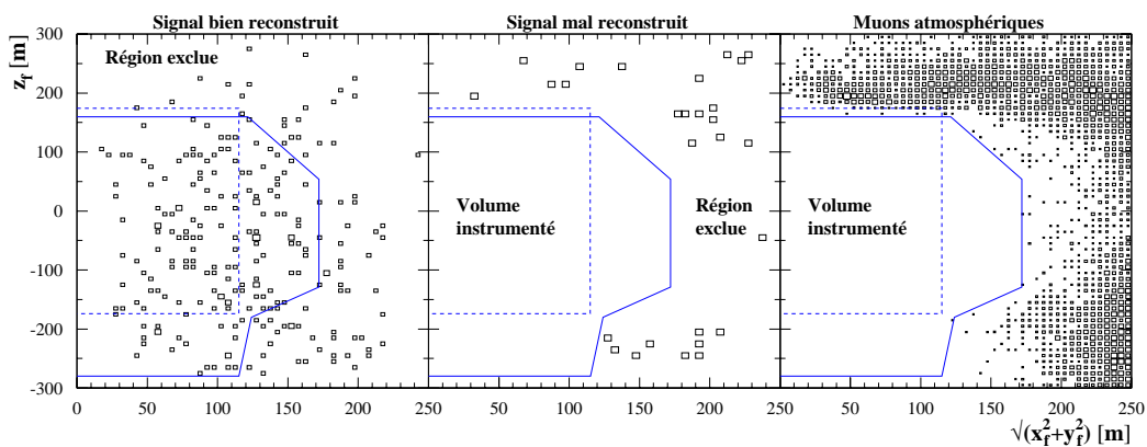
(a) Événements reconstruits ascendants
