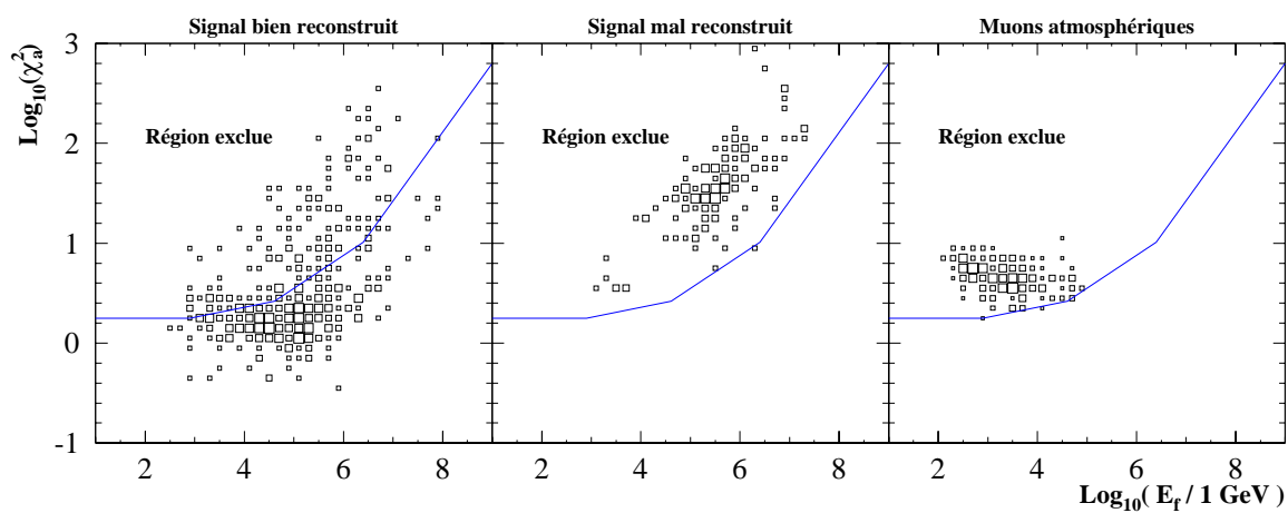
Figure 5.9: Distributions de \chi_a^2 pour les événements du signal bien reconstruits, mal reconstruits, et pour les événements du bruit de fond dû aux muons atmosphériques. La présélection et toutes les autres coupures sont appliquées.
