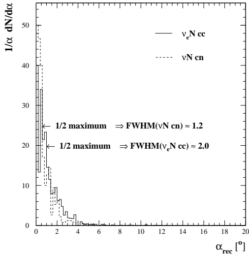
Figure 5.22: Distribution de l'erreur angulaire globale, pondérée par 1/\alpha_{rec} pour être proportionnelle à la densité d'événements par unité d'angle solide (équation 5.2, voir texte).
