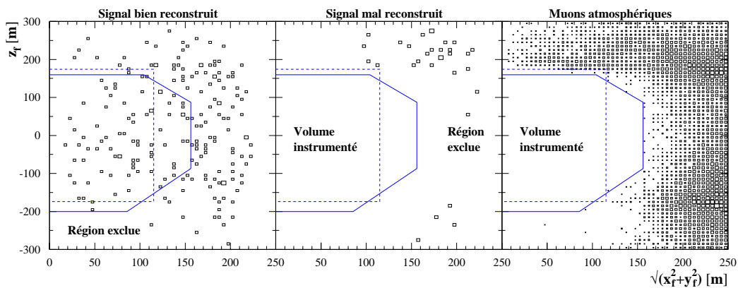
(b) Événements reconstruits descendants
