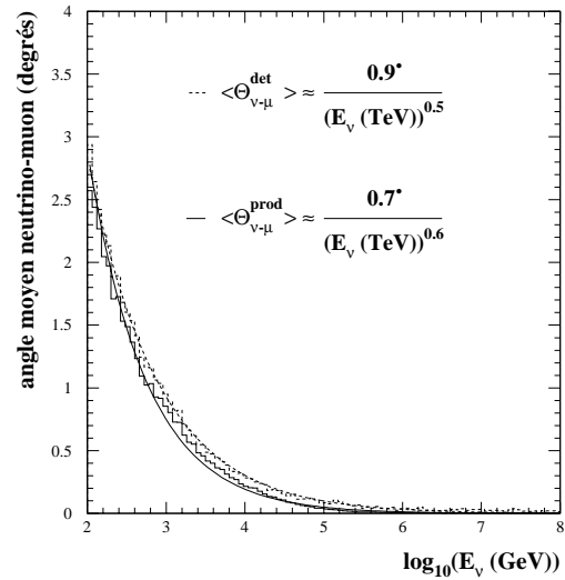
Figure 2.4: Angle moyen entre le neutrino et le muon produit (traits pleins) ou le muon lorsqu'il arrive au détecteur (pointillés). La courbe en pointillés tient compte des diffusions multiples dans la roche, ce qui dégrade légèrement la corrélation.
