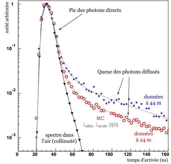
Figure 3.8: Distributions des temps d'arrivée sur un photomultiplicateur des photons issus d'une source pulsée située à 24 m (cercles) ou 44 m (étoiles). La même expérience dans l'air (triangles) sert de témoin. Les courbes représentent les ajustements de la simulation dont sont extraits les paramètres optiques de l'eau.
