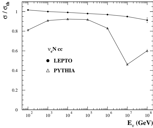
Figure 4.4: Rapport des sections efficaces totales calculées par simulation (LEPTO ou PYTHIA) ou par intégration numérique ( \sigma_{th} ), pour le processus \nu_e N cc .
