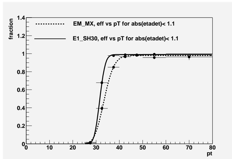
FIG. 5.1 – Efficacités des triggers utilisés.
