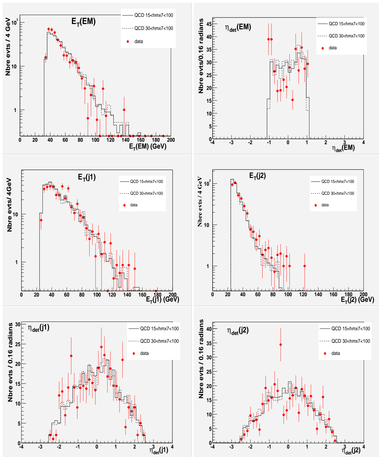
FIG. 5.6 – Distributions cinématiques pour le “DATA sample” et “QCD sample” à \cancel{E}_t < 10 GeV. Un autre “QCD sample” y est représenté, défini pour 30 < hmx7 < 100 .
