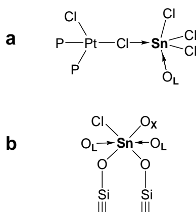
Figure 4. 45 : spectroscopie EXAFS au seuil de l'étain : espèce riche en chlore (a) et riche en oxygène (b). O_L : ligand oxygène de type L (acétone, silanol ou eau) ; O_X : ligand oxygène de type X (hydroxy, silanolate)
