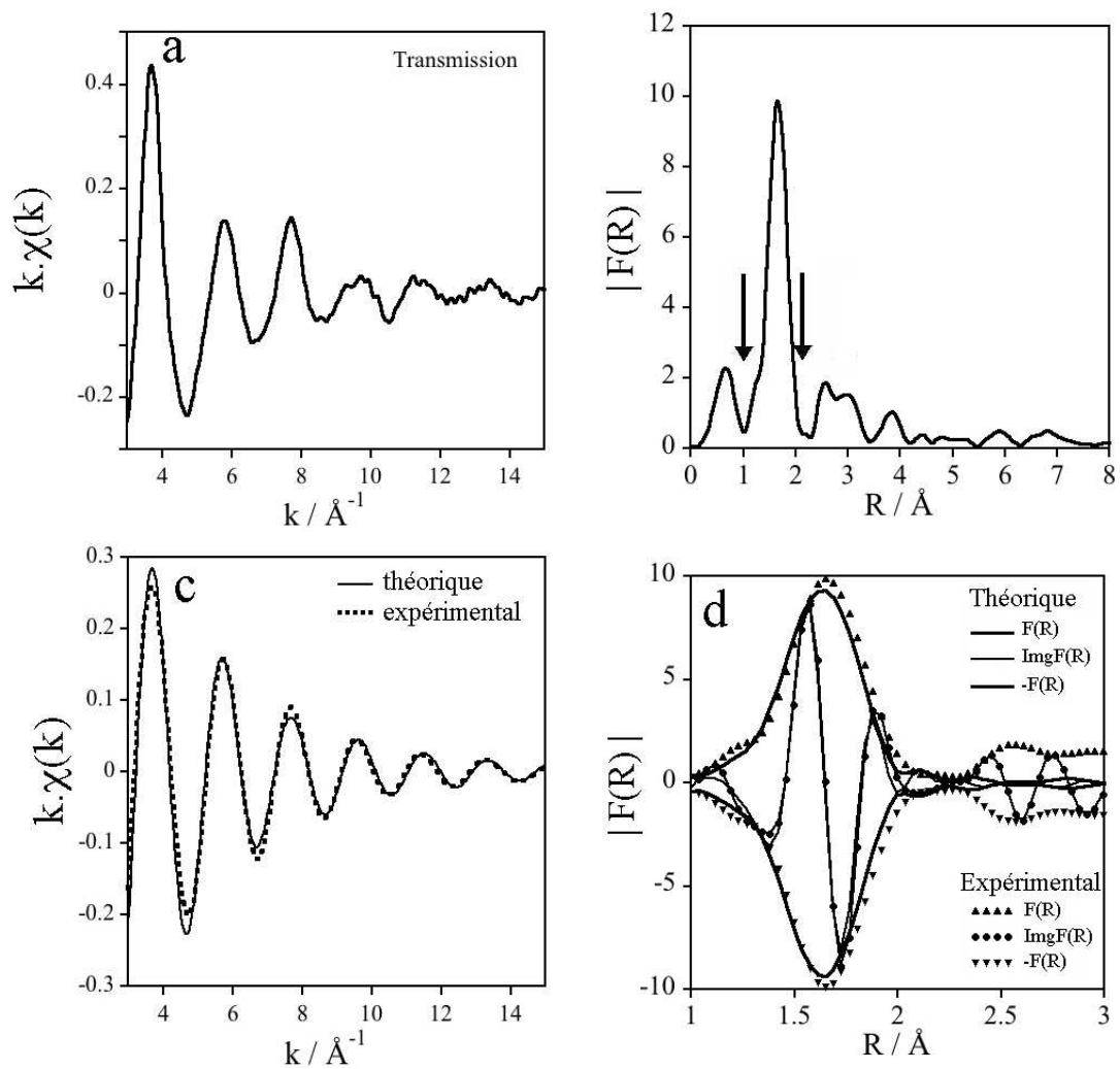
Figure B. 5 : EXAFS du complexe \text{Pt}(\text{acac})_2 ; a : oscillations entre 3 et 15 \text{\AA}^{-1} (bruit = 0,014) ; b : transformée de Fourier calculée avec une fenêtre de type Kaiser ( \tau = 3,0 ) ; c : filtre de transformée de Fourier du signal expérimental pris entre 1,00 et 2,09 \text{\AA} et simulation avec d_{\text{Pt-O}} = 197 \text{ pm} et \sigma_{\text{O}}^2 = 21 \text{ pm}^2 ; d : transformée de Fourier inverse du filtre et de la simulation.
