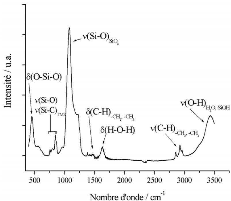
Figure 2. 7 : Spectre IR d'un matériau de type LUS-AS .
