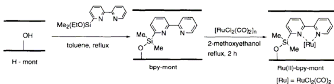
Figure 1. 17 : Immobilisation d'un complexe de Ru(II) dans la montmorillonite [91] .
