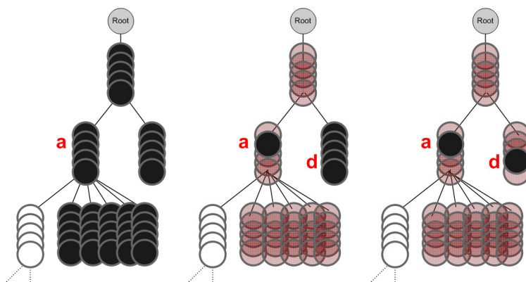
FIG. 5.8: Nouveau principe de maximalité appliqué au premier AMM de la Figure 5.6 A gauche, la ligne de niveau la plus significative est trouvée. L'étiquette a correspond à l'étiquette de la Figure 5.4. Au milieu, les lignes de niveaux qui sont parents ou enfants de cette ligne de niveau sont supprimées du AMM. A droite, la ligne la plus significative suivante est à nouveau trouvée (étiquette d ). A la fin de cette étape, le AMM est vide, et l'algorithme passe au AMM suivant.
