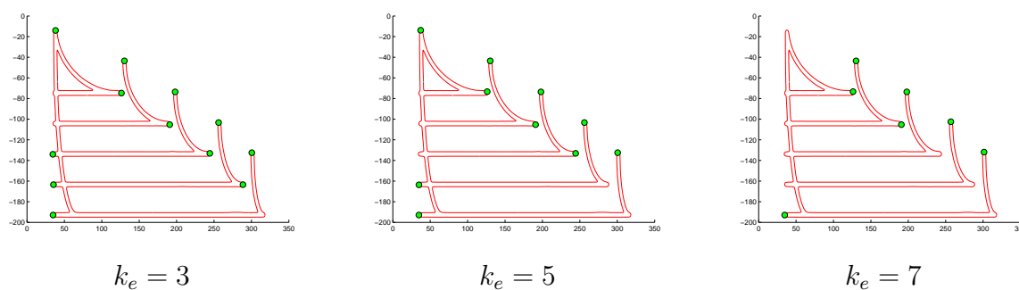
FIG. 6.19: Influence de k_e . En vert, les extrémités détectées. Augmenter k_e accroît le risque de manquer les extrémités qui sont à une distance inférieure à k_e R_\Phi d'un croisement de traits. Inversement, abaisser k_e accroît le risque de détecter certaines jonctions étirées de deux traits comme étant une extrémité.
