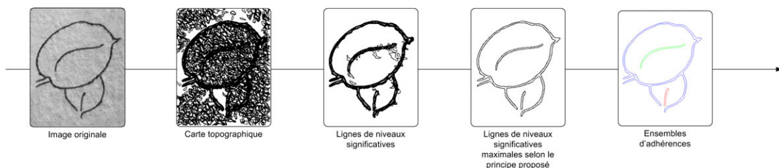
FIG. 5.10: Schéma global de la méthode proposée d'extraction des contours de traits. Tout d'abord, l'image est représentée par sa carte topographique. Le modèle probabiliste rappelé à la Section 5.2.1 est ensuite appliqué pour sélectionner les lignes significatives. Le principe de maximalité que nous avons proposé à la Section 5.3.1 élimine ensuite les lignes redondantes. Chaque agrégat de traits est enfin décrit par un ensemble d'adhérence constitué des lignes de niveaux significatives maximales décrivant ses contours. Dans ce chapitre, nos contributions à ce schéma global de détection sont les deux dernières étapes.
