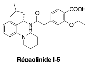
Répaglinide I-5
