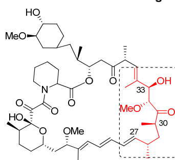
Rapamycine Schéma 87
