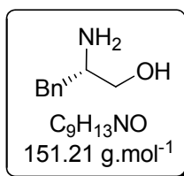
(S)-(-)-2-amino-3-phenylpropan-1-ol 197
