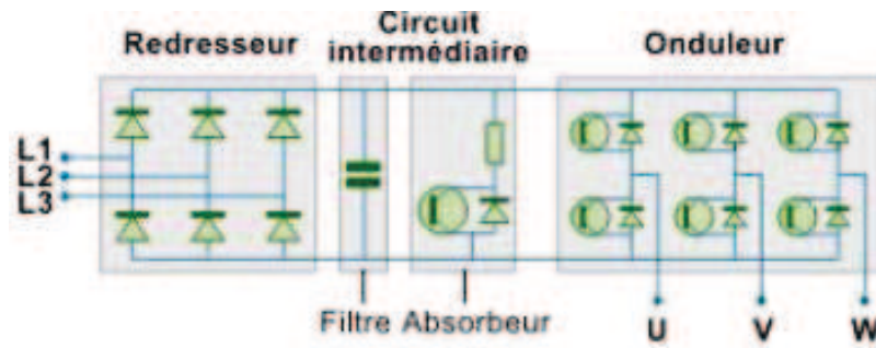
Figure 39. Composition du circuit d'électronique de puissance du variateur de vitesse
