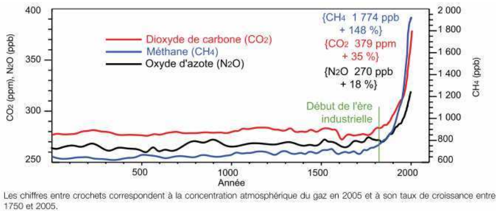
Figure 1. Evolution du taux de concentration de différents gaz à effet de serre
