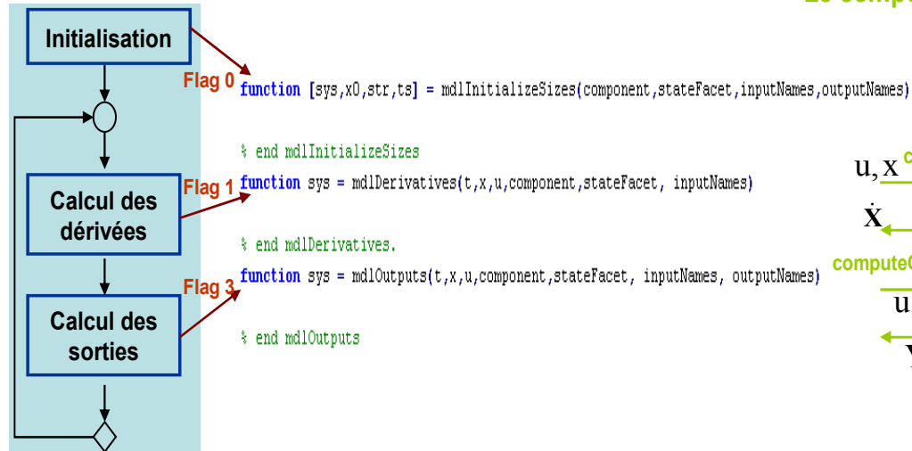
Figure 103. L’interaction entre l’ICAr encapsulé dans une S-fonction et le solveur de Matlab lors d’une simulation ODE continue
