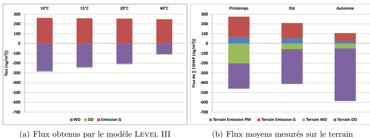
FIGURE 5.9 – Comparaison des flux à l'interface sol-air pour la somme des 15 HAP. (a) Résultats obtenus pour le modèle LEVEL III©, et (b) ceux mesurés sur le terrain.
