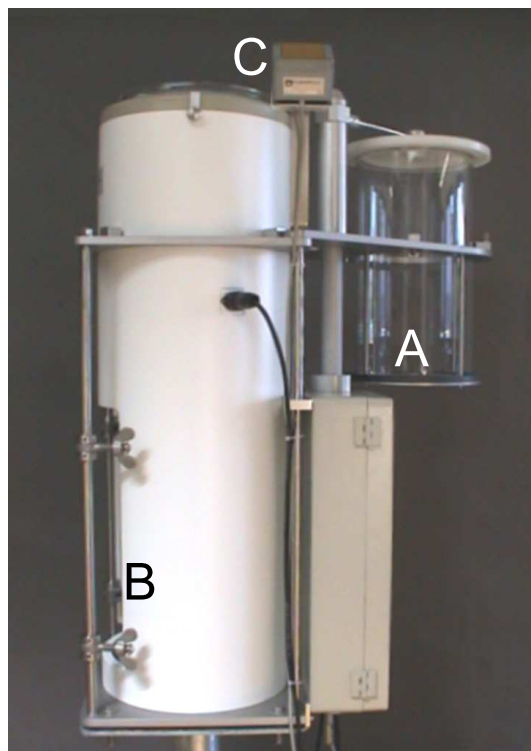
FIGURE 2.4 – Prélèvement de retombées atmosphériques sèches (DS) et humides (DH). (A) collecteur des DS, (B) collecte des DH, et (C) détecteur infrarouge
