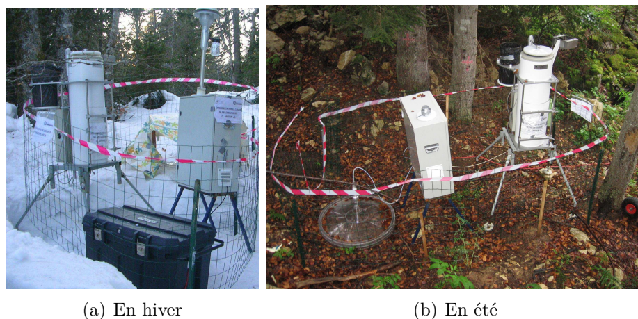
FIGURE 2.7 – Matériels mis en place sur le site de montagne. (a) en hiver, (b) en été
