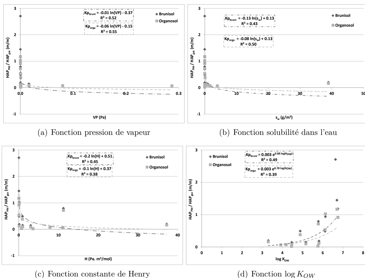
FIGURE 3.4 – Partage particules/gaz ( K_P ) en fonction des propriétés physicochimiques des HAP. (a) la pression de vapeur, (b) la solubilité dans l'eau, (c) la constante de Henry, (d) le logarithme du coefficient de partage octanol-eau
