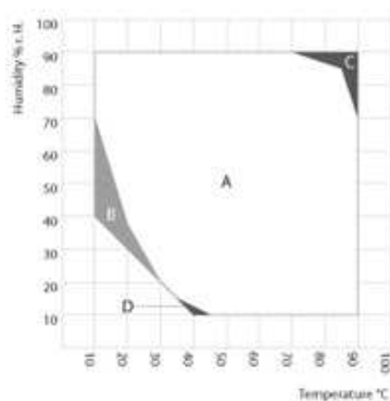
FIGURE 2.2 – Diagramme des conditions de travail en température & humidité contrôlées de la chambre climatique KMF240. (A) Utilisation normale, (B) possible sur une courte période (<24h) et (C & D) pas de garantie de stabilité.
