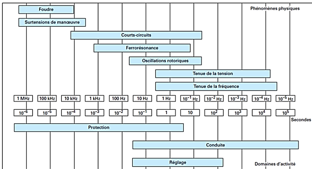
Figure 1-2. Echelles temporelles des différents phénomènes physiques dans un réseau (Source : (Meyer & al., 1998))
