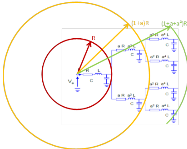
Figure 3-3. Méthode de croissance d'une boule appliquée au réseau de Cantor.
