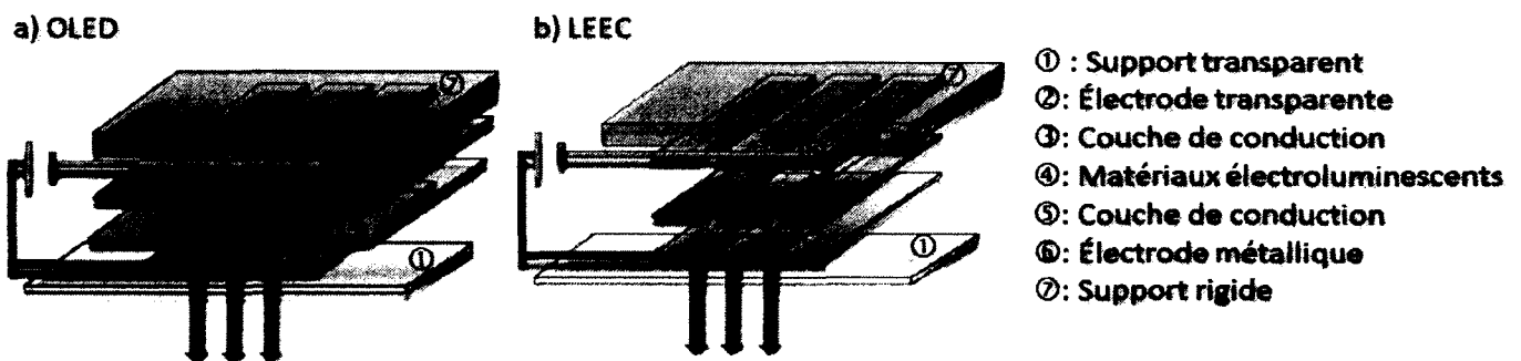
Figure 12. Structure schématique a) d'une OLED et b) d'une LEEC.
