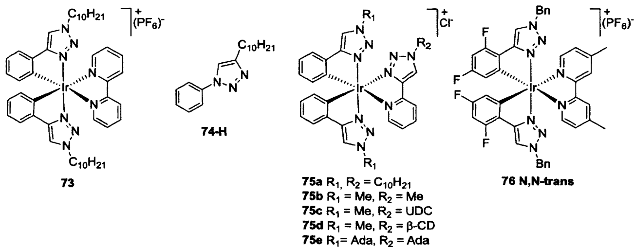
Figure 33. Exemples des complexes portant des ligands cyclométalliques contenant des unités 1,2,3-triazoles (UCD = acide ursodésoxycholique, \beta -CD = \beta -cyclodextrine et Ada = adamantyle).
