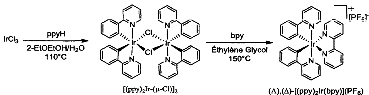
Schéma 1. Voie classique de synthèse des complexes de type [(ppy) 2 Ir(bpy)](PF 6 ).
