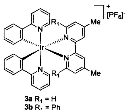
Figure 15. Complexes synthétisés par M. Lepeltier et coll. et leurs propriétés photophysiques dans l'ACN à 298 K et EtOH/MeOH (4/1) à 77 K. 55
