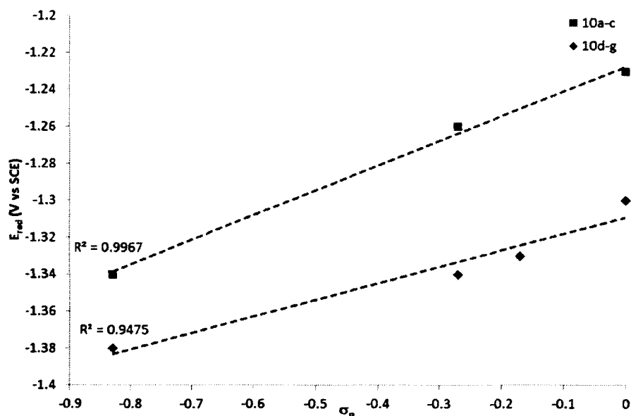
Figure 24. Déplacement du potentiel de réduction du ligand N N dans les complexes 10a-g en fonction du paramètre de Hammett ( \sigma_p ).
