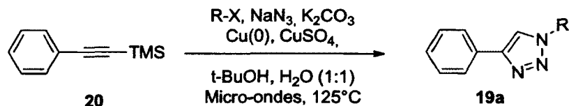
Schéma 6. Conditions typiques expérimentées par François Mathieu (R-X est MeI ou BnBr et R = Me ou Ph respectivement).
