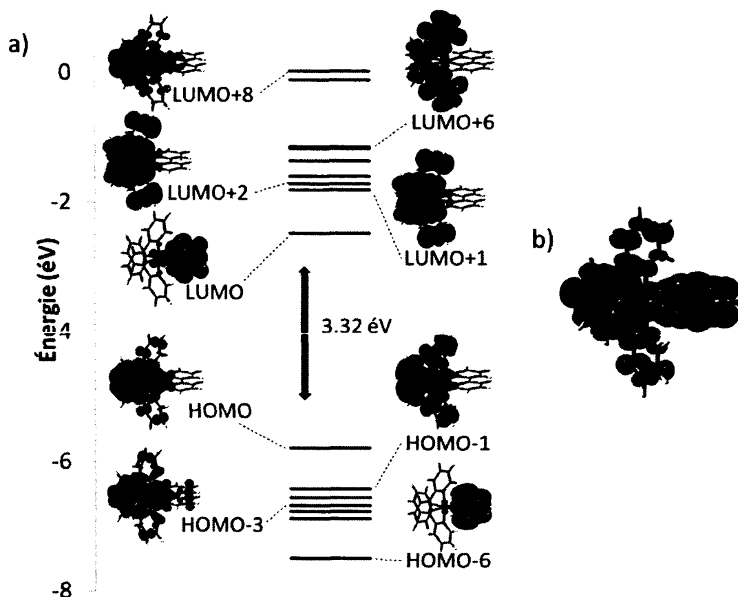
Figure 8. a) Diagramme de Kohn-Sham des OMs de LUMO+8 à HOMO-6, incluant les images des OMs d'intérêts (isodensité 0.02) calculées par DFT du complexe 1. b) Représentation de la densité de spin à l'état triplet (isodensité 0.0004) du complexe 1.
