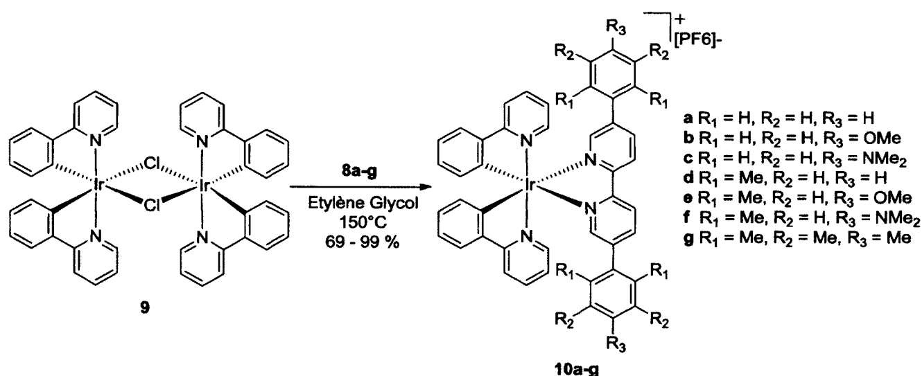
Schéma 3. Synthèse des complexes 10a-g .
