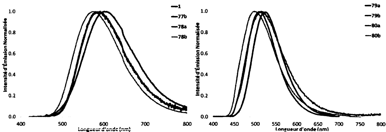
Figure 39. Spectres d'émission en solution dans l'ACN à 298 K des complexes 1 , 77b à 80a-b .
