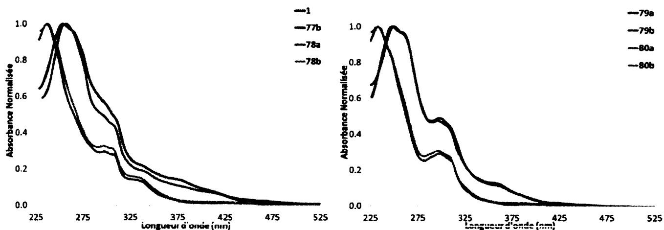
Figure 37. Spectre d'absorption en solution dans l'ACN à 298 K des complexes 1, 77b à 80a-b.
