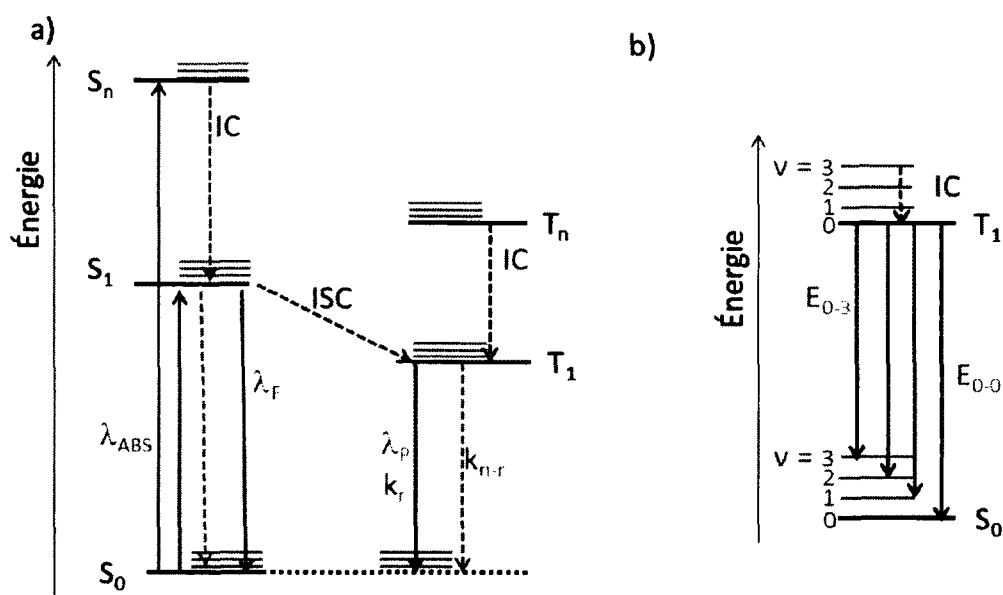
Figure 2. a) Diagramme de Jablonski montrant les transitions d'absorption (mauve), les conversions internes (IC, rouge) et le croisement inter-système (ISC, rouge), les transitions non-radiatives (orange), radiatives (bleu) et les états vibrationnels (vert). b) Agrandissement montrant l'origine des bandes d'émission possédant des états vibrationnels excités.
