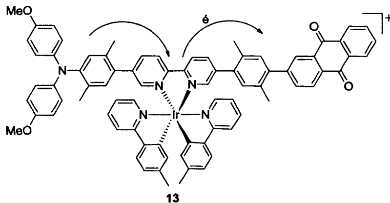
Figure 30. Système biaisé électroniquement synthétisé par le groupe de Hankache et coll. 69
