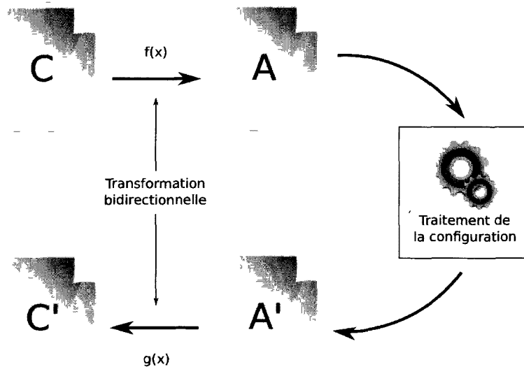
FIGURE 2 – Étapes de transformation d'un fichier de configuration
