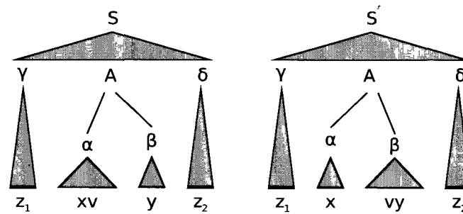
FIGURE 2.10 – Arbres syntaxiques résultant d'une ambiguïté horizontale
