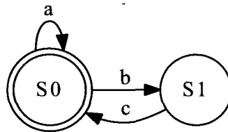
FIGURE 2.2 – Machine à états finie du langage (a|bc)^*
