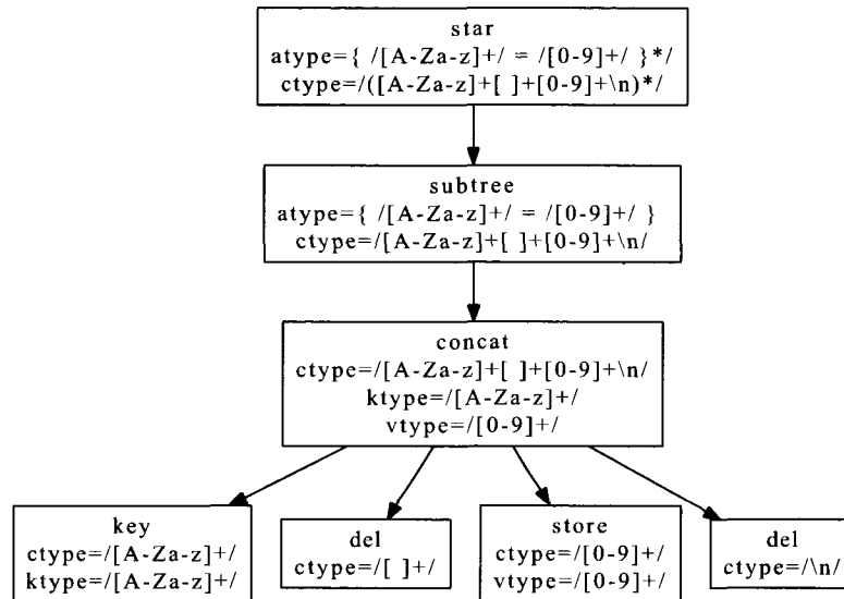
FIGURE 4.4 – Hiérarchie de la lentille record
