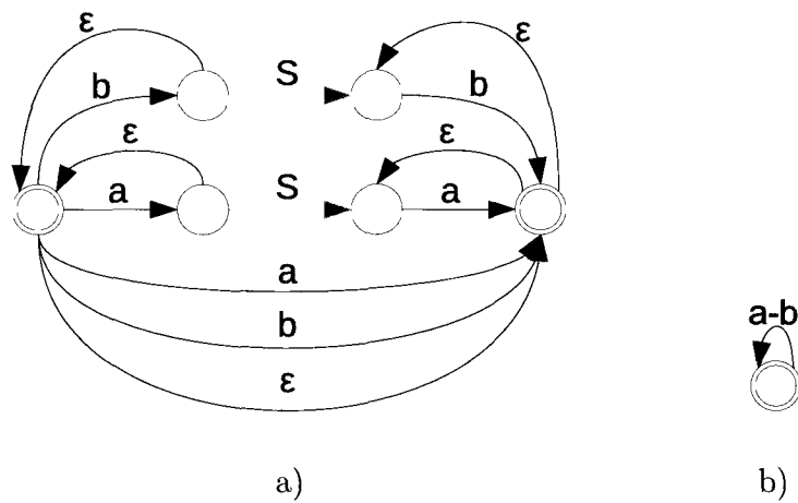
FIGURE 2.6 – RTN de la grammaire de l'exemple 2.3.1
