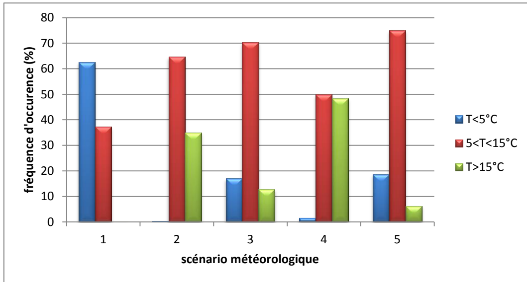
Figure 32 : Distribution des températures sur les différents scénarios météorologiques
