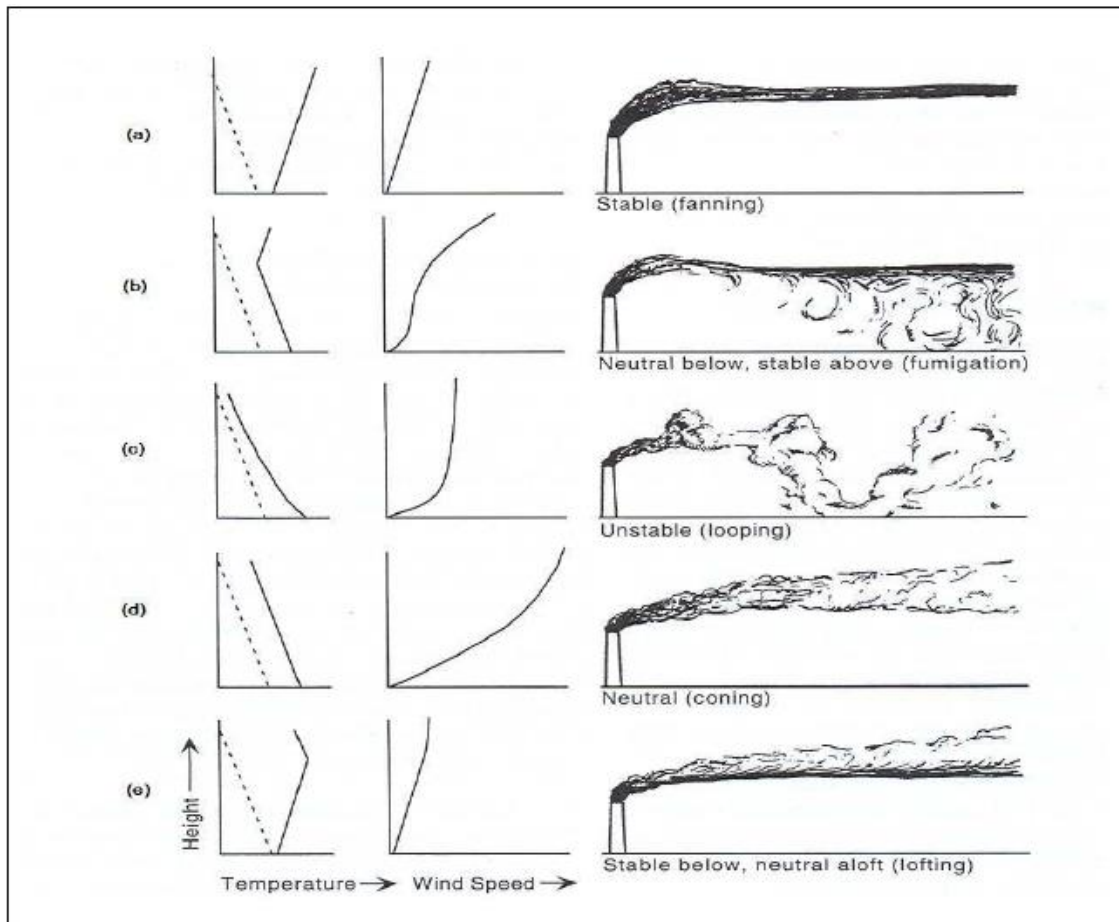
(a) : Panache horizontale (fanning) ; (b) : Panache d'enfumage (fumigation) ; (c) : Panache sinueux (looping) ; (d) : Panache conique (coning) ; (e) : Panache tourmenté vers le haut (lofting)
