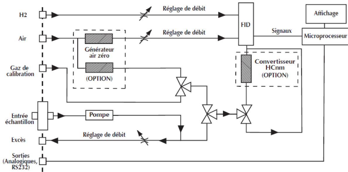
Figure 23 : Schémas du fonctionnement de l'analyseur on-line HC51M
