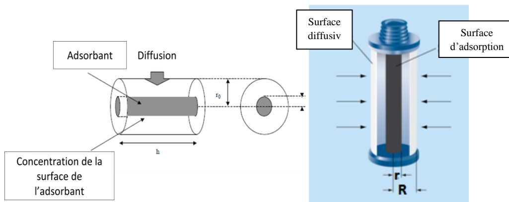
Figure 6 : Principe du prélèvement passif et schémas d'un préleveur Radiello r : rayon du tige adsorbant et R : rayon du corps diffusive
