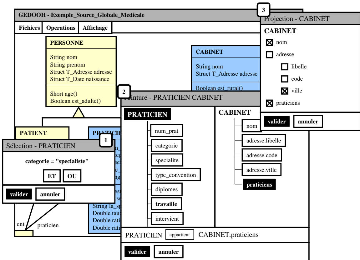
Figure 55 : Elaboration de la fonction d'extraction des cabinets médicaux.
