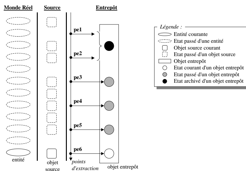
Figure 23 : Modélisation d'un objet entrepôt.
