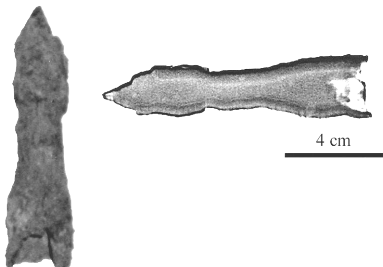
Coupe longitudinale
