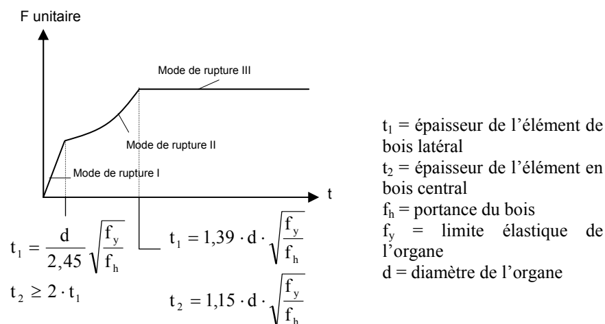
Figure A.15 : Représentation graphique du modèle de Johansen pour des assemblages bois-bois en double cisaillement avec f_{h1} = f_{h2} = f_h et M_y = d^3 \cdot f_y / 6
