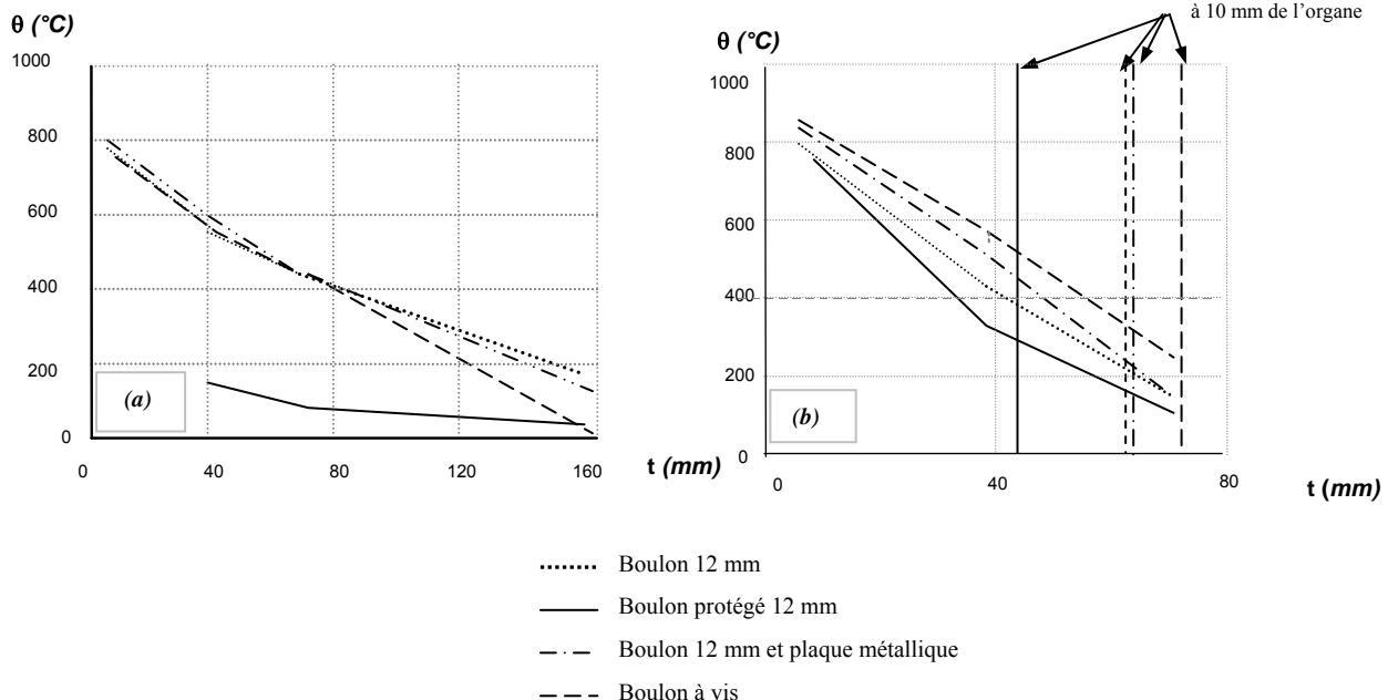
Figure A.42 : Évolution de la température dans les boulons (a) et le bois (b) pour une exposition de 90 min
