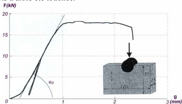
Figure A.9 : Comportement expérimental d'enfoncement parallèle au fil du bois pour de l'Epicéa ( d=20 \text{ mm} ) [BOC 97]
