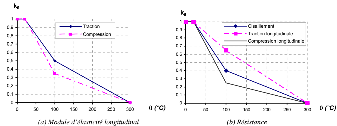
Figure A.46 : Evolution des propriétés physico-mécaniques du bois [EU52 02]
