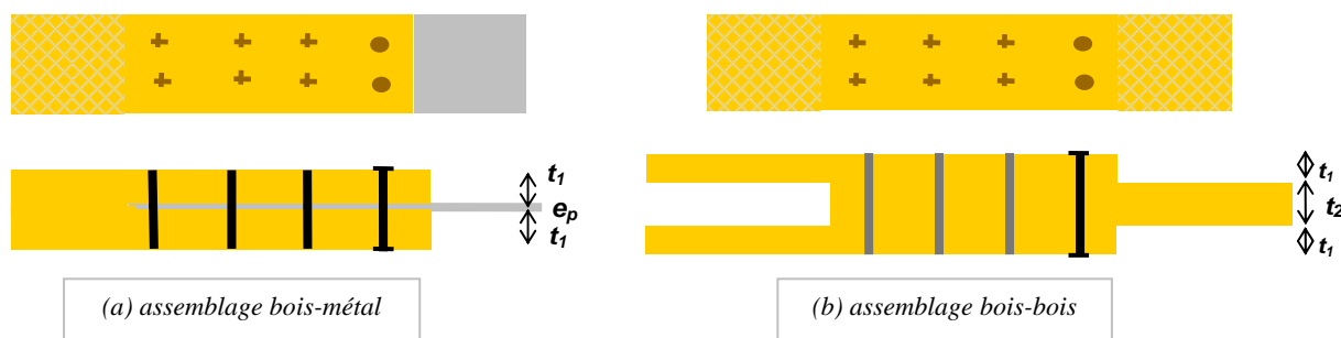
Figure C.1 : Description géométrique des assemblages
