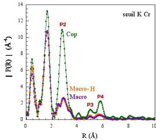
Figure IV.13 – Module de la transformée de Fourier au seuil K du Cr de la phase Zn_2Cr macroporeuse. Les distances ne sont pas corrigées des déphasages atomiques
