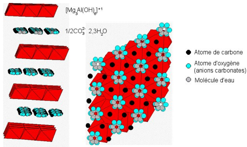
Figure III.5 – Structure de la phase \text{Mg}_3\text{Al}(\text{OH})_6(\text{CO}_3^{2-})_{0.5}, 2,3\text{H}_2\text{O} déterminée suite à l'affinement
