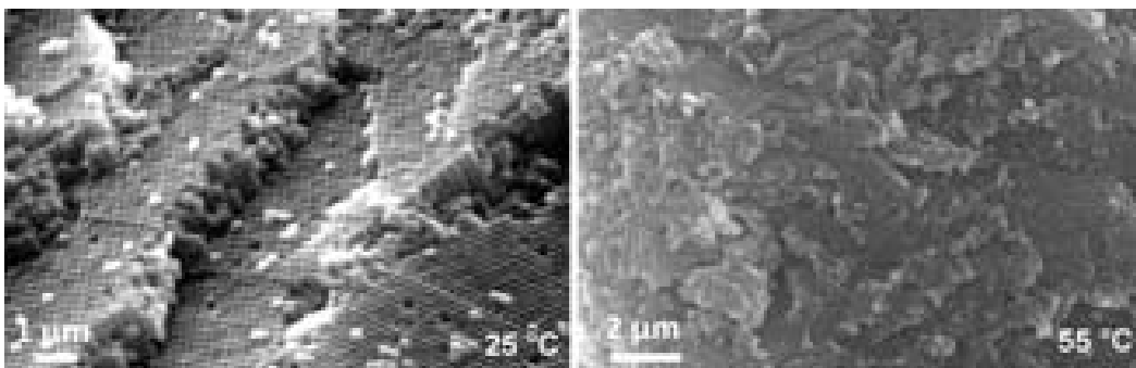
Figure II.13 – Clichés MEB de dépôts obtenus par évaporation (1%w, \phi=250 nm). 25 °C à gauche, 55 °C à droite
