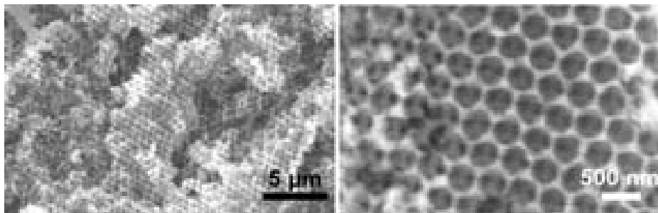
Figure II.37 – Micrographies MEB à différents grossissements des oxydes mixtes macroporeux après calcination de l’empreinte de PS
