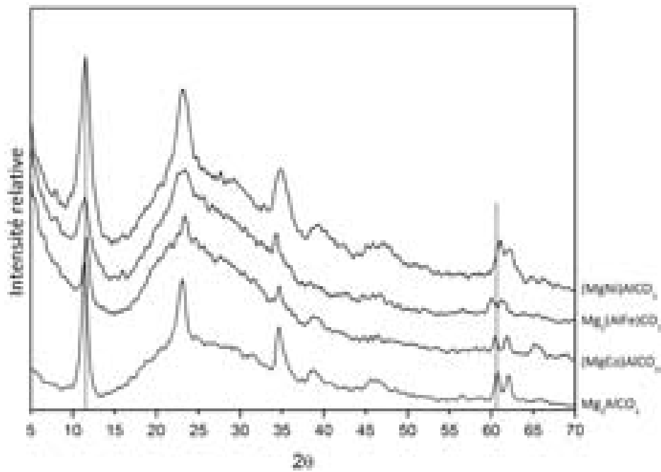
Figure IV.3 – Diffractogrammes des rayons X des phases de compositions mixtes Mg-M-Al-CO_3
