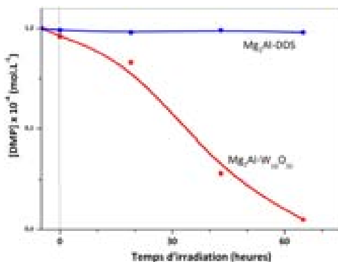
Figure V.17 – Activités photocatalytiques des phases MgAl macroporeuses intercalées par l'anion DDS ou l'anion decatungstate
