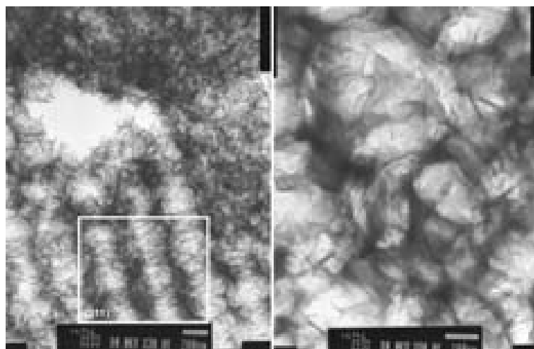
Figure II.38 – Clichés de microscopie électronique à transmission des oxydes mixtes macroporeux à différentes magnitudes
