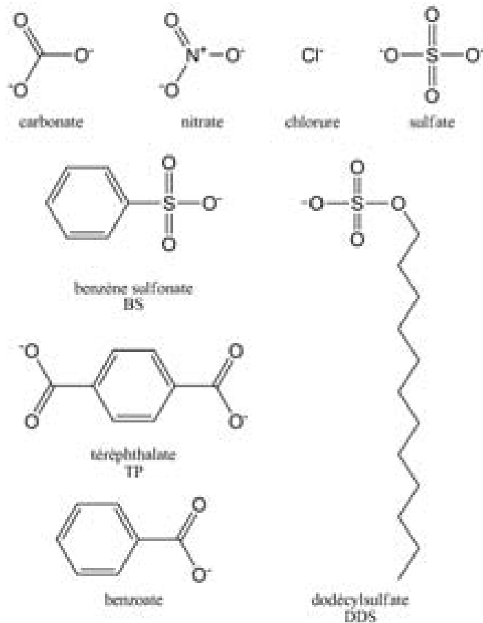
Figure III.9 – Structure des différents anions étudiés
