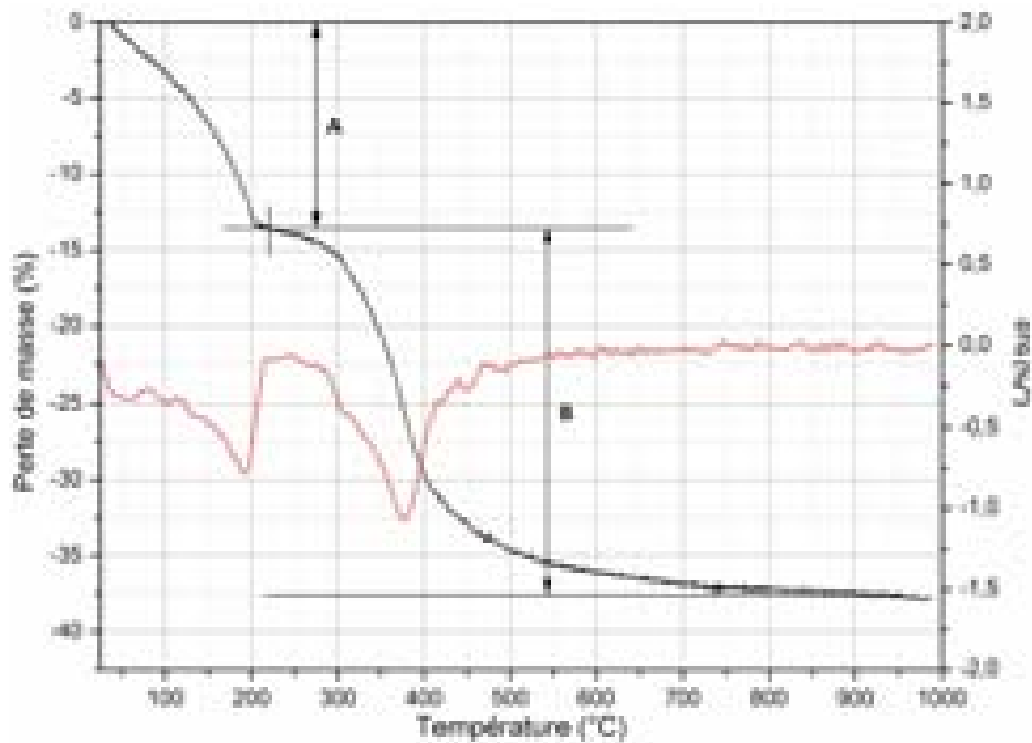
Figure III.19 – Analyse thermogravimétrique de la phase Mg_2Al macroporeuse de 25 °C à 1000 °C
