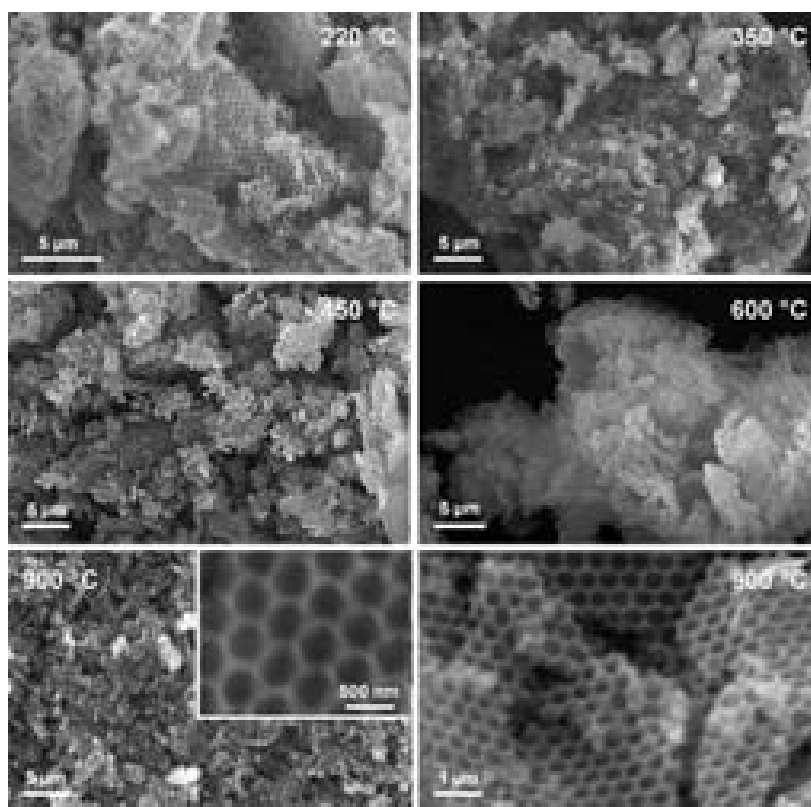
Figure III.22 – Images de microscopie électronique à balayage de la phase macroporeuse Mg_2Al-CO_3 en fonction de la température
