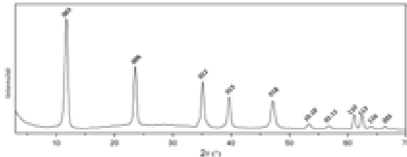
Figure I.21 – Diffractogramme des rayons X d'une phase Mg_2Al-CO_3
