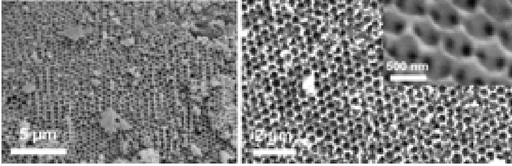
Figure II.43 – Micrographies MEB des phases HDL macroporeuses reconstruites sous air humide (50 %) (gauche) et dans l'eau (droite) après calcination de l'empreinte de PS ( \phi_{billes}=600 nm)
