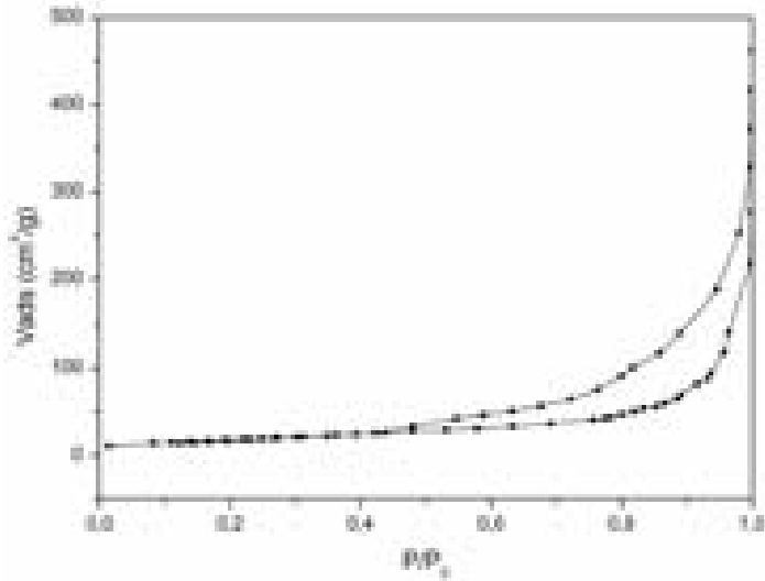
Figure II.48 – Isotherme d'adsorption d'une phase Mg_2Al macroporeuse obtenue après élimination de l'empreinte par calcination
