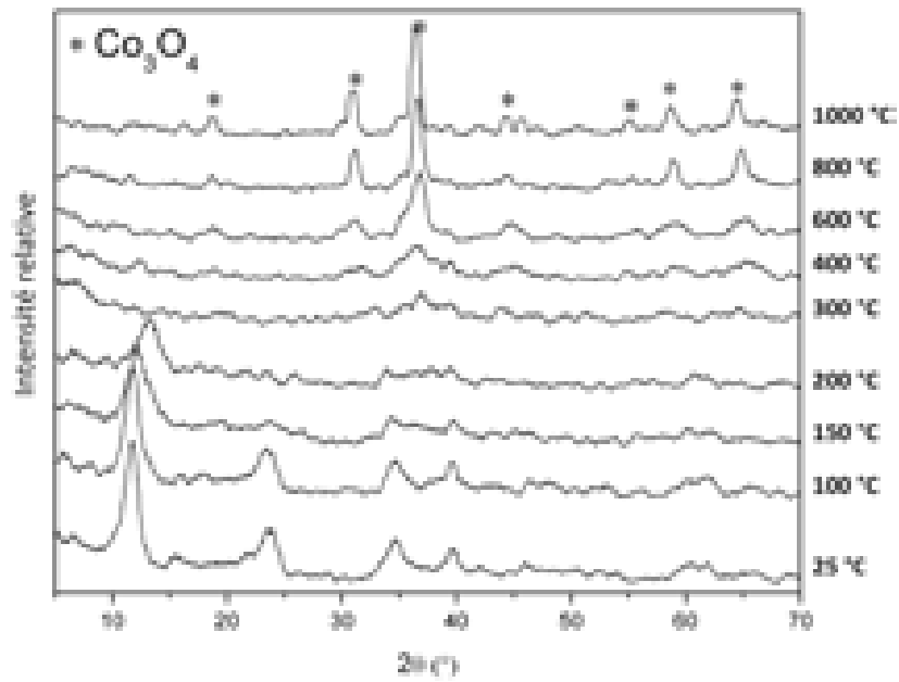
Figure IV.17 – Étude par diffraction des rayons X in-situ de la phase \text{Co}_2\text{Al} macroporeuse en fonction de la température
