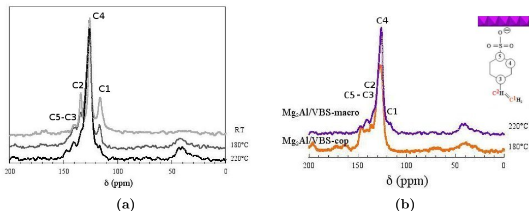
Figure V.27 – Spectres ^{13}C CP-MAS RMN d'une phase macroporeuse Mg-Al-VBS après traitements thermiques à 180 °C et à 220 °C (a), et comparaison des spectres d'une phase macroporeuse Mg-Al-VBS après traitement thermique à 220 °C et d'une phase Mg-Al-VBS « classique » après traitement thermique à 180 °C (b)
