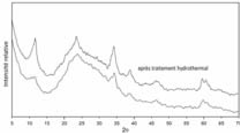
Figure IV.2 – Diffractogrammes des rayons X de la phase Zn_2Cr avant et après traitement hydrothermal
