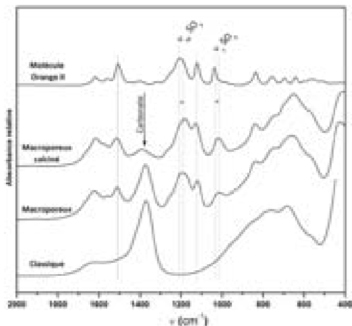
Figure V.5 – Spectres infrarouge des phases Mg_2Al « classique » et macroporeuse et leurs oxydes mixtes obtenus suite à une calcination à 420\text{ °C} , après les isothermes d'adsorption, comparés avec le spectre du colorant Orange II
