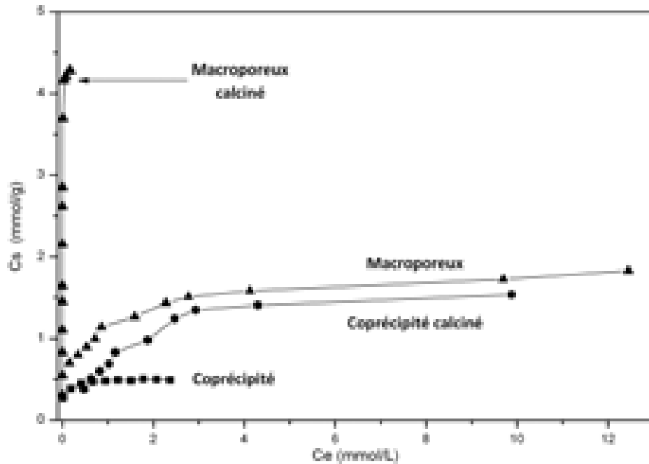
Figure V.3 – Isothermes d’adsorption du colorant Orange II pour les phases Mg_2Al macroporeuses et « classiques » et leurs oxydes mixtes respectifs obtenus suite à une calcination à 420\text{ °C}
