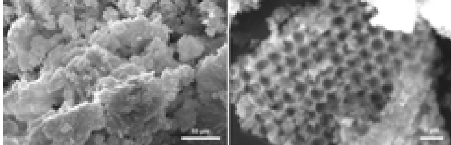
Figure III.16 – Micrographies de MEB de la phase MgAl macroporeuse traitée à reflux dans l'éthanol
