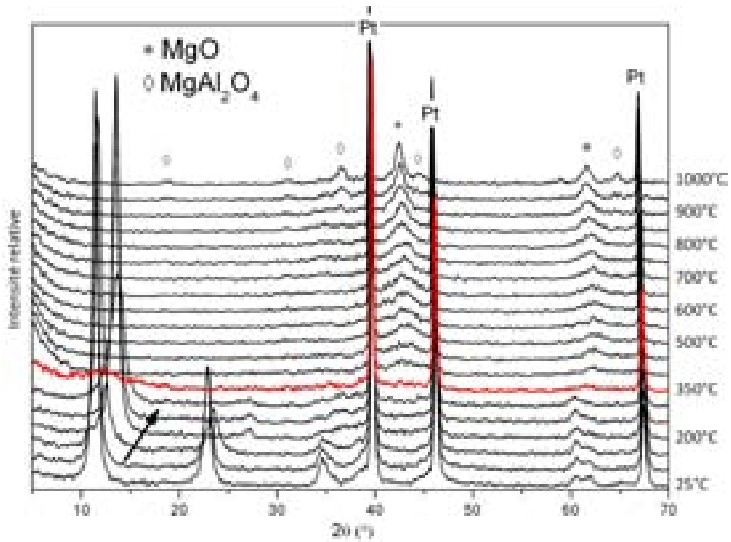
Figure III.20 – Diffractogrammes des rayons X de la phase macroporeuse Mg_2Al-CO_3 en fonction de la température
