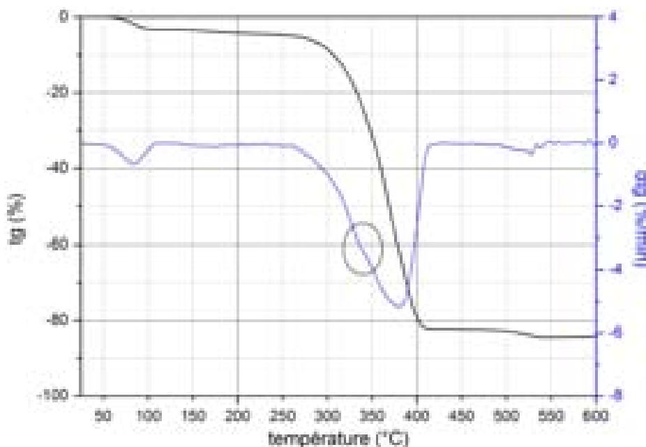
Figure II.33 – Analyse thermogravimétrique d'une opale de polystyrène de 25 °C à 600 °C
