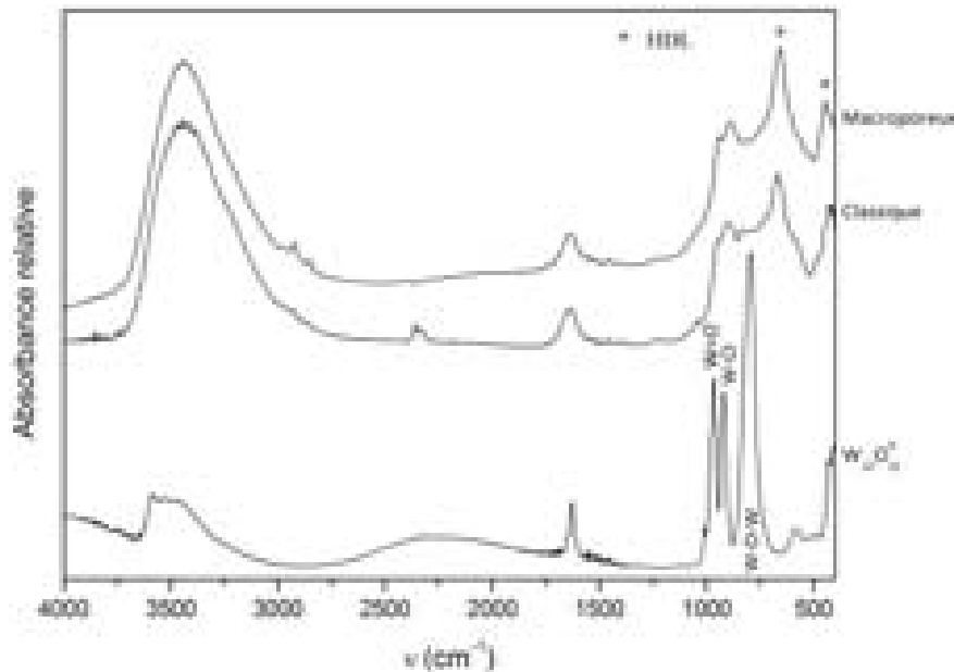
Figure V.15 – Spectres infrarouge des phases macroporeuse et classique intercalées par l'anion décatungstate
