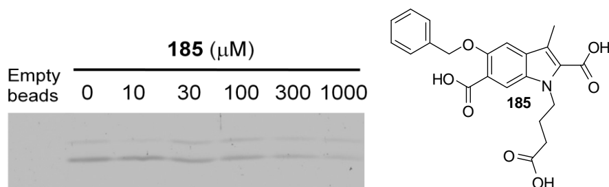
Figure 87 : Gel de chromatographie d'affinité de 185 .
