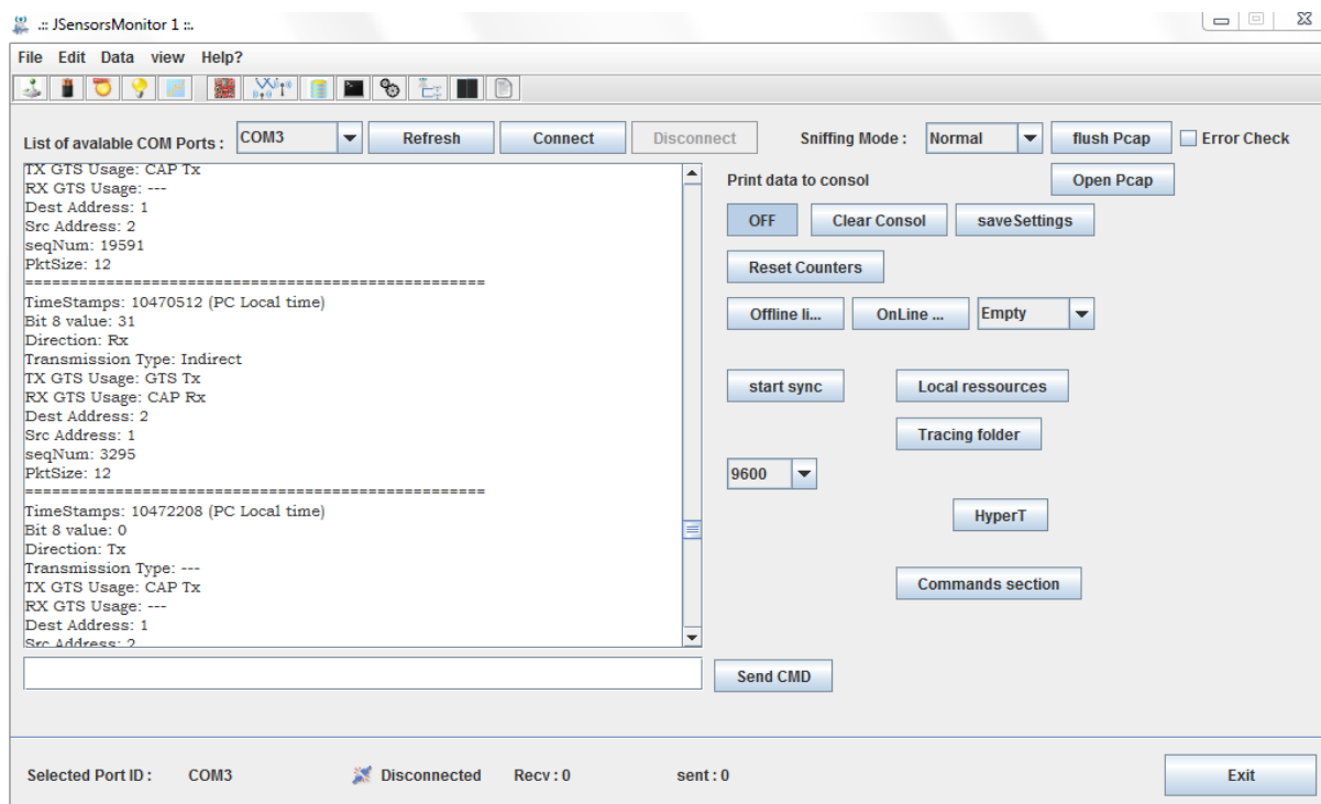
Figure 27 : Interface principale du logiciel « JSensorsMonitor »
