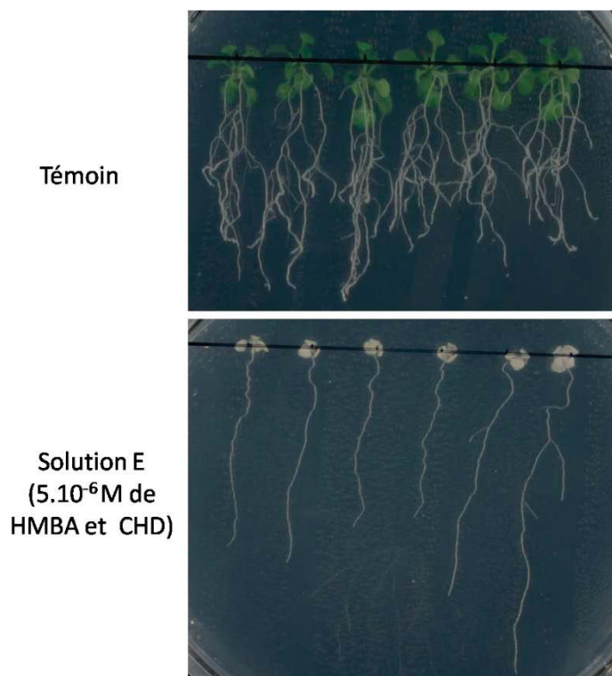
Figure 43 : Influence d'une solution de XDD totalement hydrolysé sur la croissance racinaire d' Arabidopsis thaliana . La solution E est testée pour 5 \cdot 10^{-6} M de HMBA et CHD pendant 20 jours de traitement. Un témoin de croissance est représenté à titre de comparaison.
