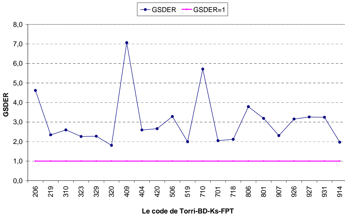
Figure 84. Variation du critère GSDER pour les couplages du tableau 30 sélectionnés parmi les couplages des 32 Torri-BD-FPTs avec les 7 Ks-FPTs de catégorie II (d'après les 6 valeurs de R_w mesurées pour 6 échantillons du site n°12).
