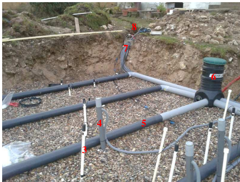
Figure 33. A-1. Etat de l'instrumentation le 20 décembre 2011. A-2. Installation d'une plaque poreuse. B. Etat de l'instrumentation le 20 janvier 2012 : 1. Le sable de granulométrie normalisée. 2. Le collecteur des tubes connectés aux plaques poreuses déjà enfouies. 3. Une canne de tensiomètre. 4. Un tube de réservation pour une sonde de teneur en eau. 5. Un tuyau d'épandage des eaux usées prétraitées. 6. La boîte de répartition. 7. Le regard pour regrouper les tubes en téflon et les câbles. 8. Le départ de la tranchée d'aménée des tubes et des câbles vers les pompes et la centrale d'acquisition dans la cave.
