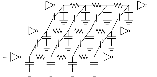
Figure 1: Modèle complet \pi 3 pour 3 fils avec couplage crossstalk .
