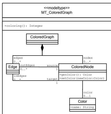
FIGURE 7.4 – Type de modèles MT_{ColoredGraph} .
