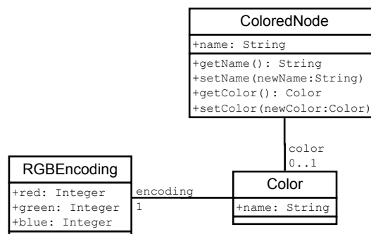
FIGURE 7.3 – Groupe de types objets ColoredNode' , Color' et RGBEncoding' .
