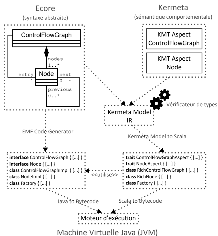
FIGURE 8.1 – Flot de compilation de l’environnement de développement de langages de modélisation dédiés Kermeta.
