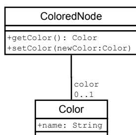
FIGURE 7.2 – Groupe de types objets ColoredNode et Color .
