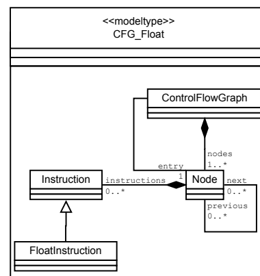
FIGURE 7.8 – Type de modèles CFG_{Float} de graphes de flot de contrôle contenant des instructions flottantes.
