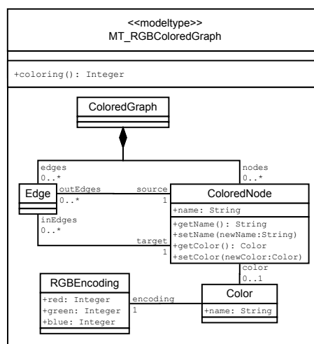
FIGURE 7.5 – Type de modèles MT_{RGBColoredGraph} .
