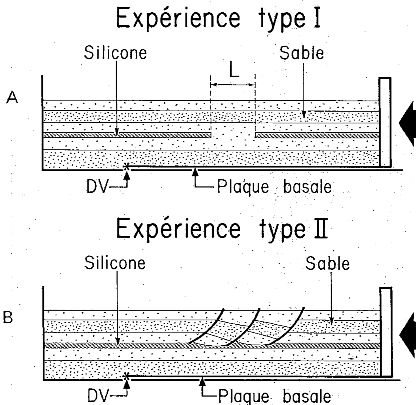
Fig. 2. — Dispositif expérimental. A. Expériences avec discontinuité du niveau ductile. L : longueur de la discontinuité. DV : discontinuité de vitesse. B. Expériences avec blocs basculés dans la couverture.
