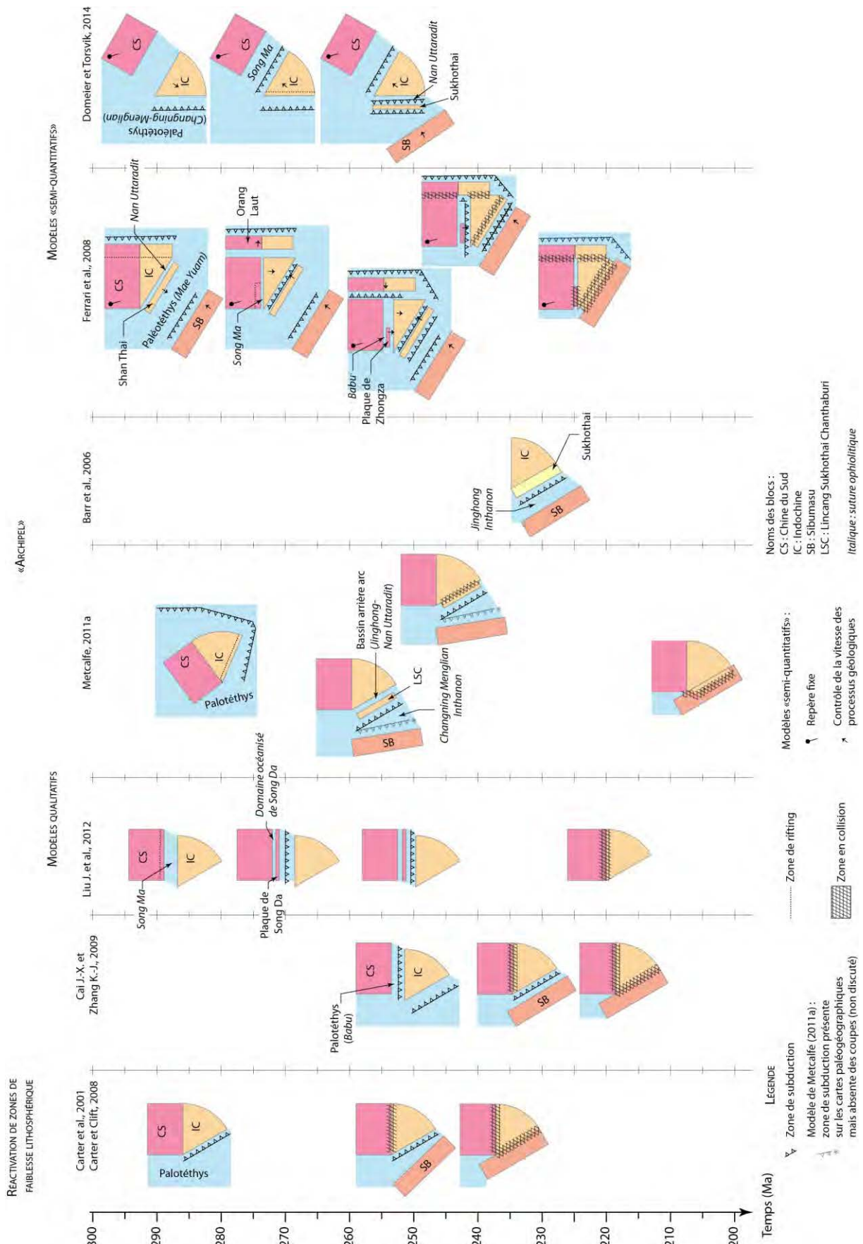
Figure 1.20. Comparaison de quelques modèles d'évolution géodynamique du domaine Est Téthysien au Permien et au Trias.
