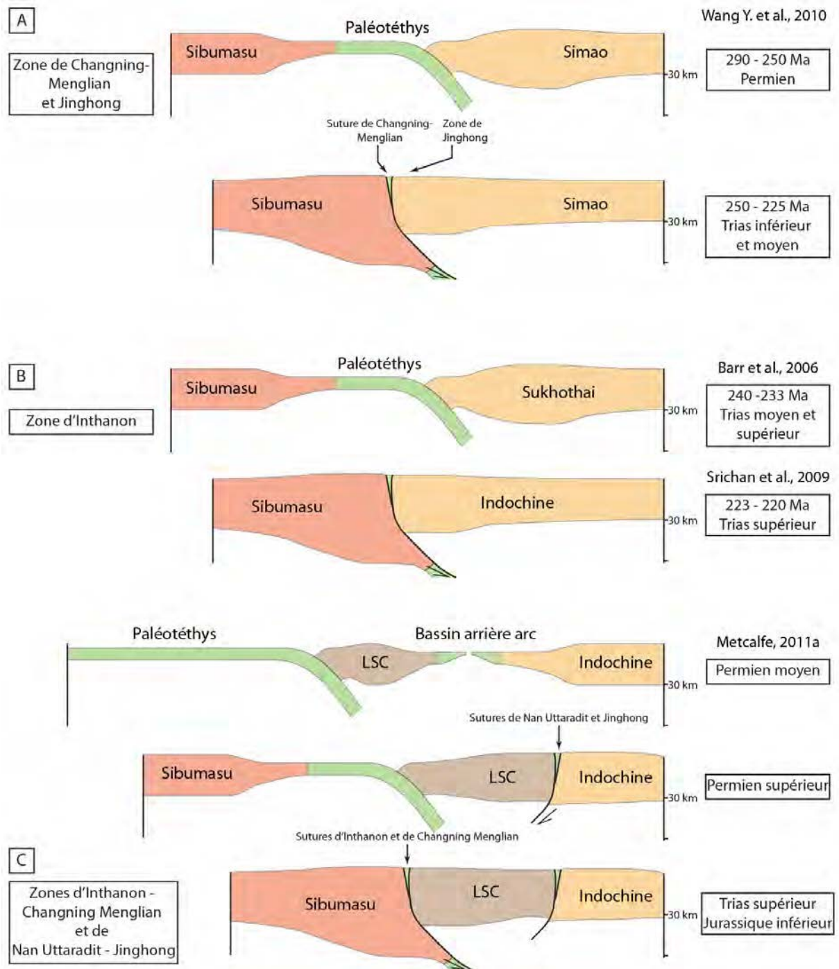
Figure 5.6. Principaux modèles d'évolution géodynamiques proposés pour les zones de Changning Menglian, Jinhong, Inthanon et Nan Uttaradit.
