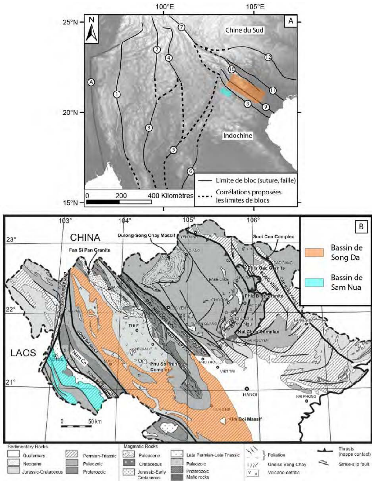
Figure 4.1. Localisation des bassins de Sam Nua et Song Da dans le domaine Est Téthysien. A. Cadre régional. A : ceinture métamorphique de Mogok, 1 : Mae Yuam, 2 : Changning Menglian, 3 : Inthanon, 4 : Jinghong, 5 : Nan Uttaradit, 6 : Loei, 7 : Ailaoshan, 8 : Song Ma, 9 : Song Da, 10 : Ailaoshan-Fluve Rouge, 11 : Song Chay, 12 : Babu. B. Carte géologique simplifiée du Nord du Vietnam et localisation des bassins de Sam Nua et Song Da par rapport à la suture de Song Ma (modifié d'après Roger et al., 2012).
