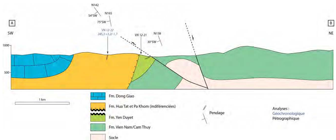
Figure 4.35. Coupe de Mai Son. Basé sur la carte révisée de la localité de Mai Son (Figures 4.22 et 4.23) selon le profil A-B (Figure 4.23).
