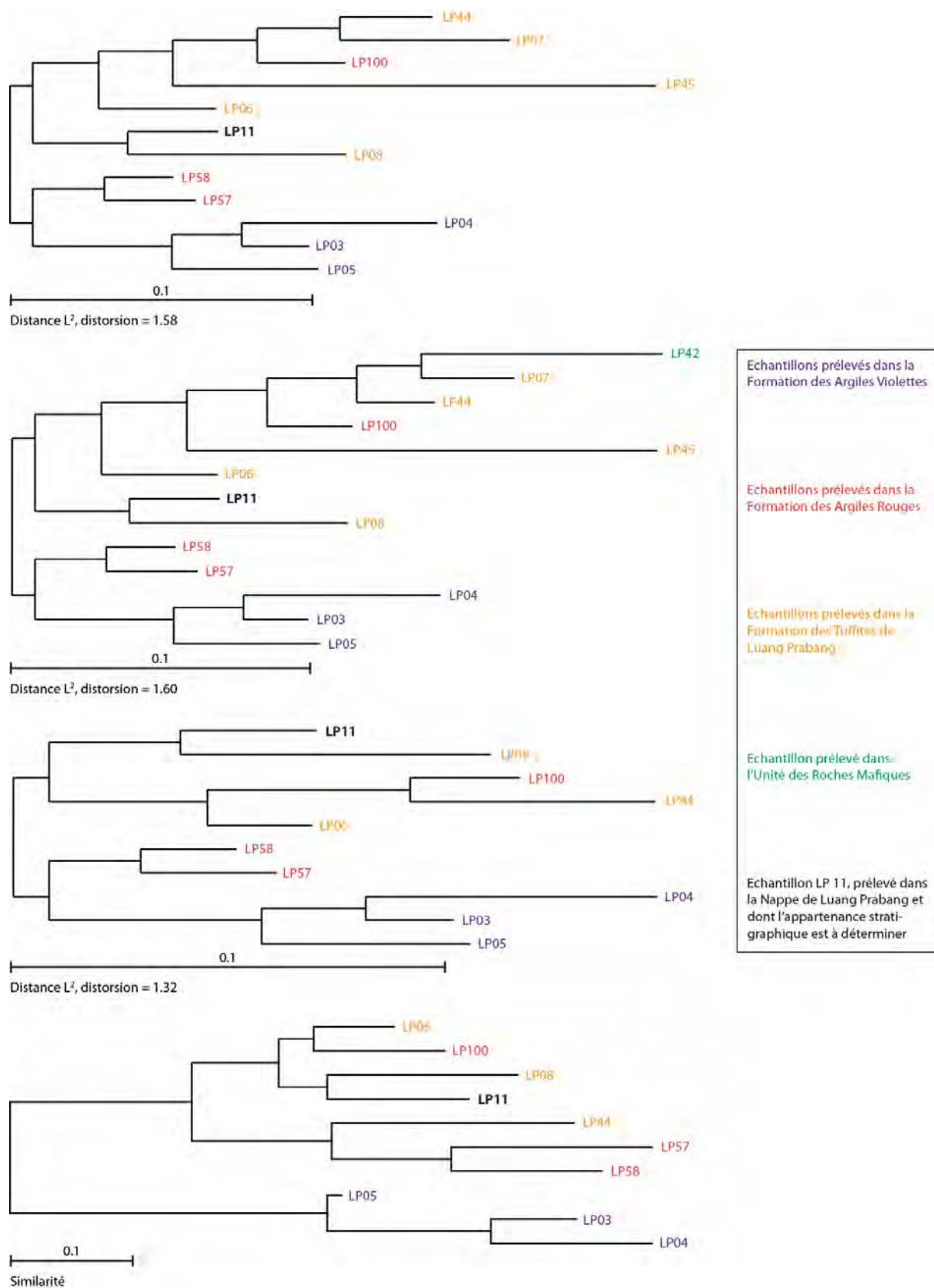
Figure 3.28. Corrélations stratigraphiques à partir des distributions d'âges. Ces arbres sont réalisés en effectuant des regroupements à partir de l'algorithme NJ. Les trois premiers arbres sont obtenus en utilisant la distance L^2 , le quatrième en utilisant la similarité.
