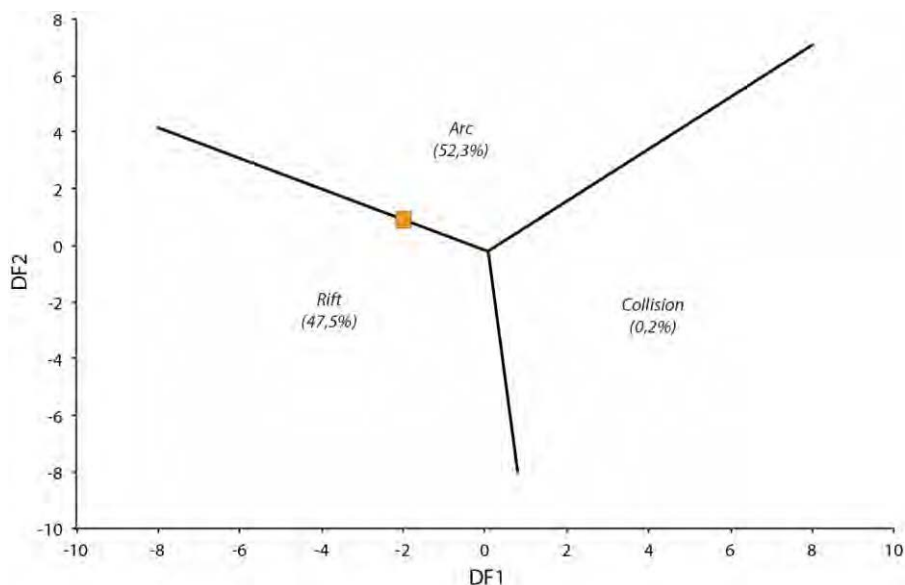
Figure 4.49. Diagramme de discrimination tectonique pour les roches sédimentaires riches en \text{SiO}_2 ( 63\% < \text{SiO}_{2(\text{adj})} \leq 95\% , Verma et Armstrong-Altrin, 2013).
