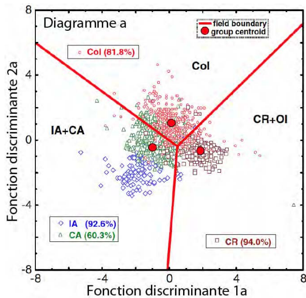
Figure 2.3. Exemple de l'un des cinq diagrammes de discrimination pour les roches acides.
