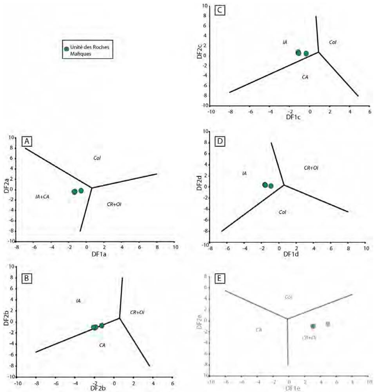
Figure 3.40. Diagrammes de discrimination des roches intermédiaires ( 52 \% < SiO_{2(adj)} \leq 63 \% ), Verma et Verma, 2013.
