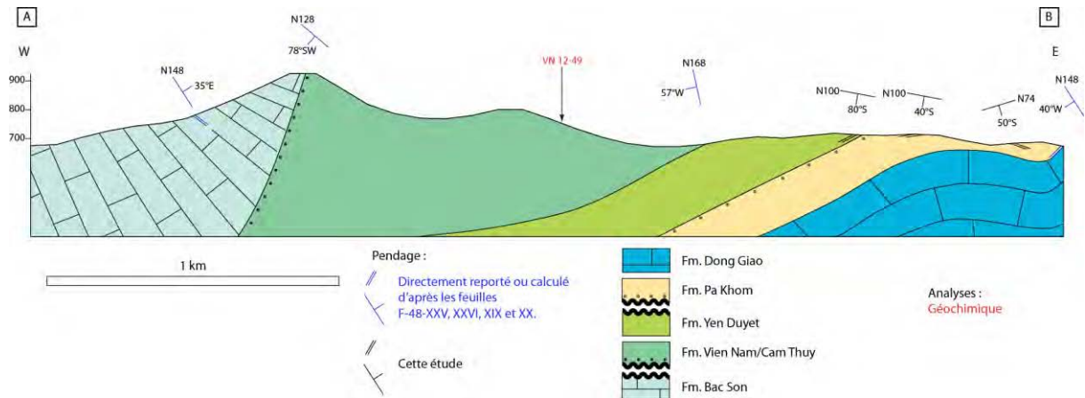
Figure 4.40. Coupe de Son La. Coupe basée sur la carte de la localité de Son La (Son et al., 2005 ; Tuyet et al., 2005 ; Figures 4.22 et 4.23) selon le profil A-B (Figure 4.23).
