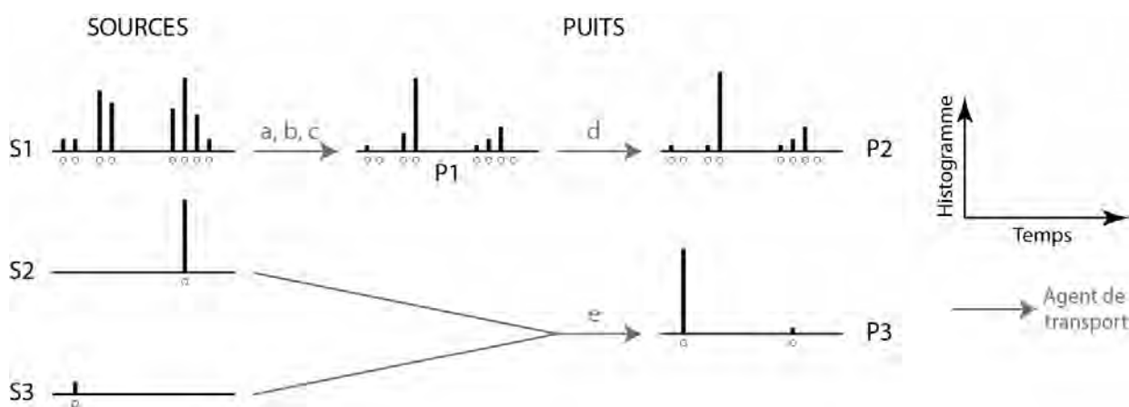
Figure 2.10. Biais liés aux processus sédimentaires et intrinsèques aux zircons.
