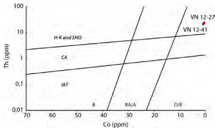
Figure 4.44 (page précédente). Diagramme Th-Co (Hastie et al., 2007) de discrimination des séries hyper-alkaline, calco-alkaline et tholéïtite d'arc.
