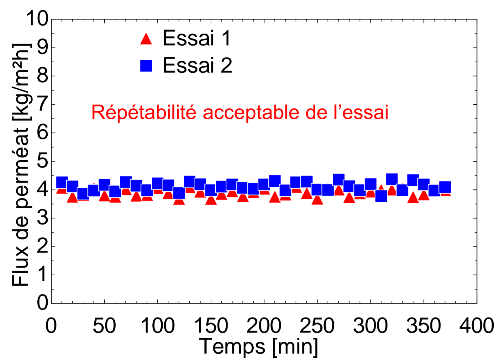
Figure 6 : Répétabilité du flux en fonction du temps ( T_c = 60^\circ\text{C} ; Q_c = 2 et Q_f = 5,25 l/min)
