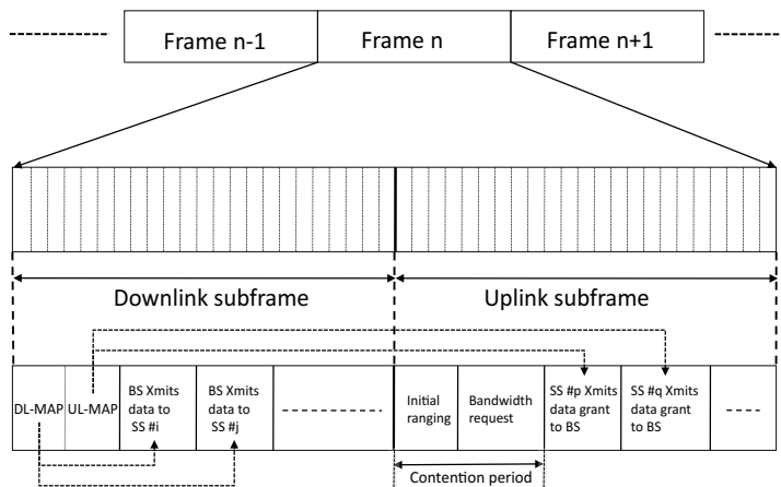
Fig. 7. IEEE802.16 MAC frame.
