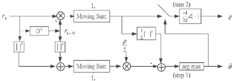
Fig. 7. The estimator (Lin, 2003)
