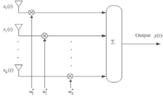
Fig. 17. Antenna beamforming
