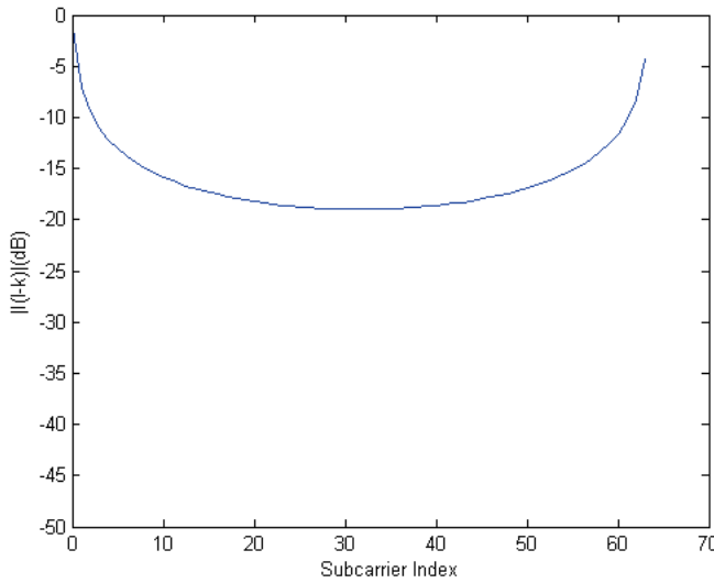
Fig. 7. ICI coefficient versus subcarrier index; N=64
