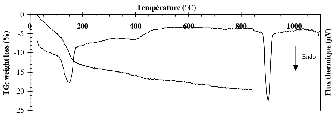
Figure B.16 : Courbes ATD-TG couplées de la birnessite KBi-700-het synthétisée à 700°C
