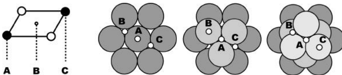
Figure 3.2 : Octaèdre MnO_6 et empilements de sphères compacts ABC
