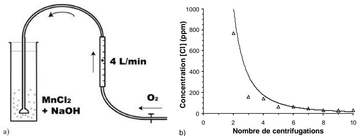
Figure 2.2 : (a) Montage expérimental lors de la synthèse et (b) évolution de la concentration en sel Cl - au cours des cycles de lavage de la busérite
