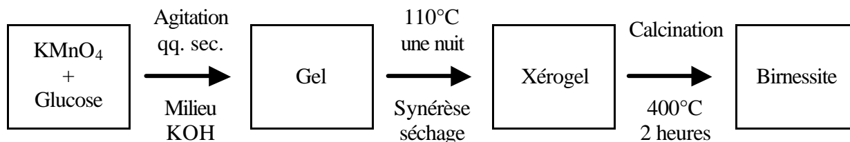
Figure 2.5 : Etapes de la synthèse de la birnessite selon le procédé sol-gel
