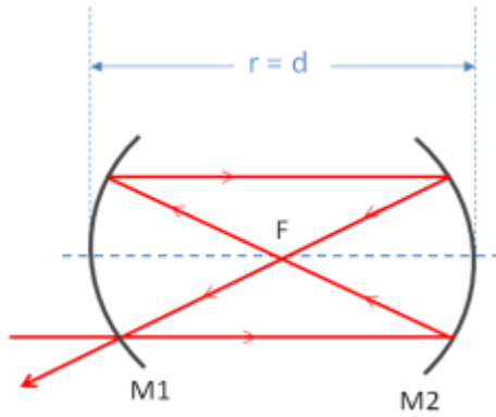
FIG. 3.6. Schématisation de l'étalon FPI 100.
