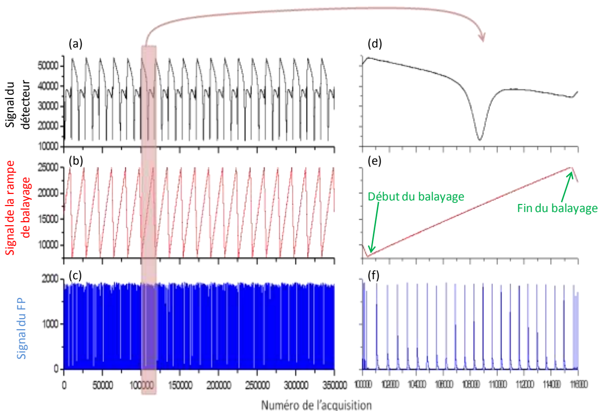
FIG 3.14. Exemple des signaux enregistrés pour la raie de CO 2 (pur) centrée à 6233,182896 cm -1 . La mesure a été faite à température ambiante et pour une pression de 150,2 Torr. Les graphes de gauche représentent (de haut en bas) le signal du détecteur avec la raie d'absorption, le signal de la rampe de balayage et enfin le signal du Fabry-Pérot. A droite, nous avons zoomé ces mêmes graphes sur une seule rampe de balayage.
