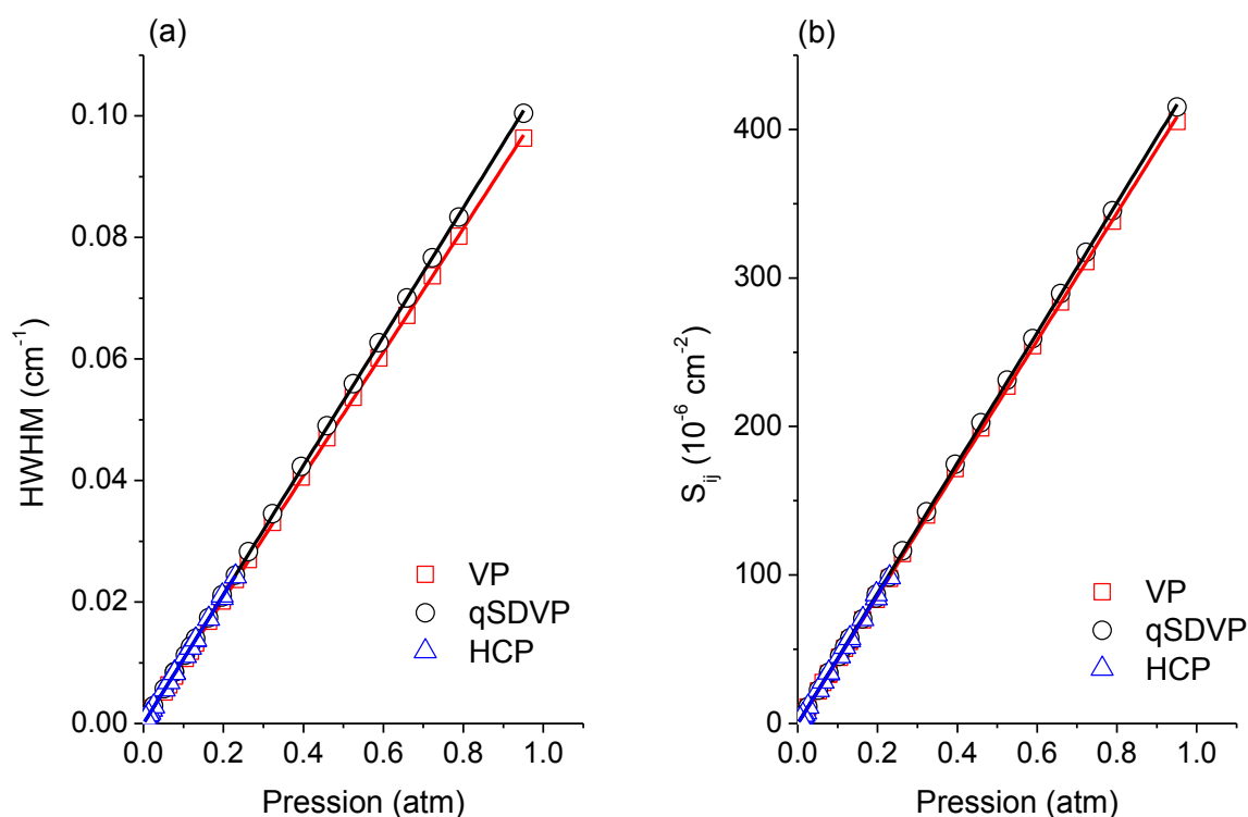
FIG. 6.2. Exemple de la détermination (a) du coefficient d'élargissement \gamma_{ij}^{auto} et (b) de l'intensité intégrée S_{ij} pour la raie R(14) de la bande (30013) ← (00001) de CO 2 pur obtenus par l'analyse spectre-par-spectre. En rouge sont représentés les résultats pour le VP, en noir ceux du qSDVP et en bleu ceux du HCP. Les coefficients d'élargissement sont directement obtenus par la pente des droites. Les intensités intégrées représentées par les pentes des droites tracées en (b) sont les intensités par unité de pression ( S_{ij}^P en cm -2 .atm -1 ).
