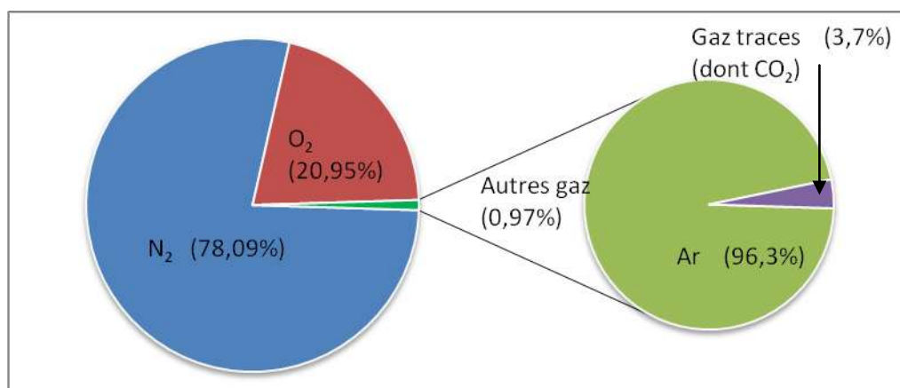
FIG. 1.1. Composition principale de l'atmosphère terrestre [Delmas 2006, Liang 2013].
