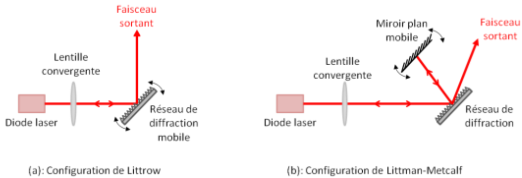
FIG. 3.3. Diode laser accordable à cavité externe (a) en configuration Littrow et (b) en configuration Littman-Metcalf.
