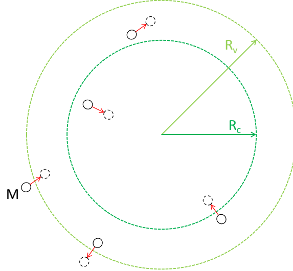
FIG 4.3. Représentation schématique de la sphère de coupure et de la sphère des plus proches voisins (sphère de Verlet en vert clair) autour d'une molécule.
