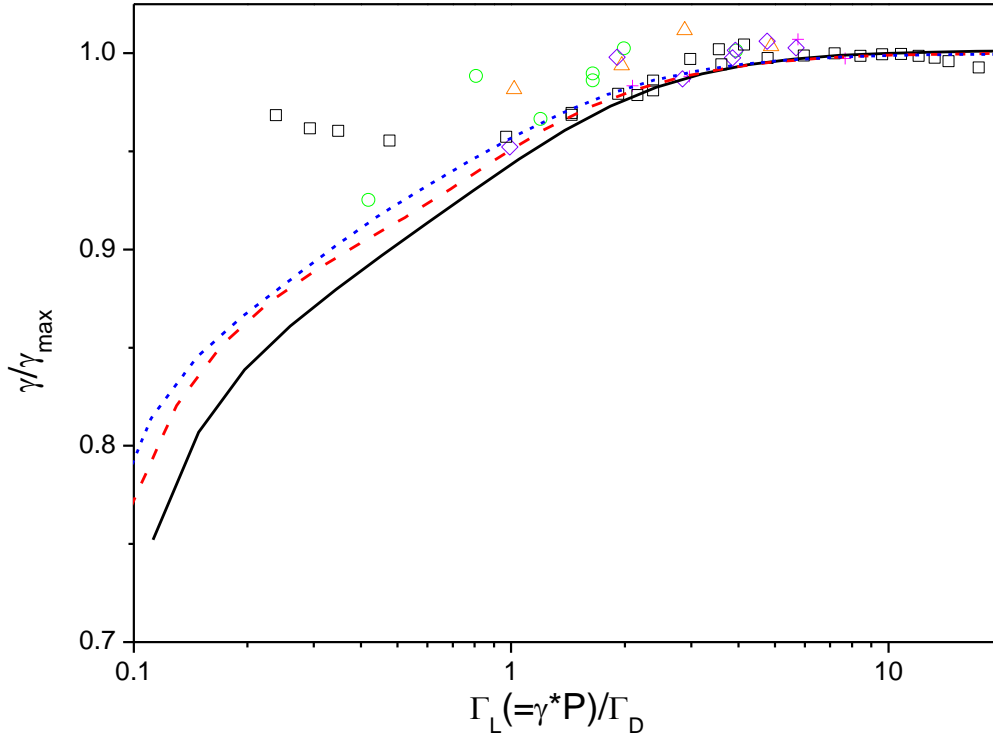
FIG. 7.13. Coefficient d'élargissement obtenus par les ajustements par le VP des spectres mesurés (points) et calculés (lignes) en fonction du rapport \Gamma_L/\Gamma_D pour la raie R(10) centrée à 6236,03699 \text{ cm}^{-1} . Les différents rapports de mélange utilisés sont représentés par les différents symboles ( \square pour le \text{CO}_2 pur, \circ pour le mélange de \text{CO}_2 à 25 % dans \text{N}_2 , \triangle pour le mélange de \text{CO}_2 à 20 % dans \text{N}_2 , + pour le mélange de \text{CO}_2 à 15 % dans \text{N}_2 , \diamond pour le mélange de \text{CO}_2 à 10 % dans \text{N}_2 et \star pour le mélange de \text{CO}_2 à 5 % dans \text{N}_2 ) pour les spectres mesurés. Les lignes en trait plein noires représentent les coefficients d'élargissement obtenus pour les spectres calculés pour le \text{CO}_2 pur, ceux pour un mélange de \text{CO}_2 à 50 % dans \text{N}_2 sont en lignes discontinues rouges et ceux pour un mélange de \text{CO}_2 infiniment dilué dans \text{N}_2 avec les lignes pointillées bleues.
