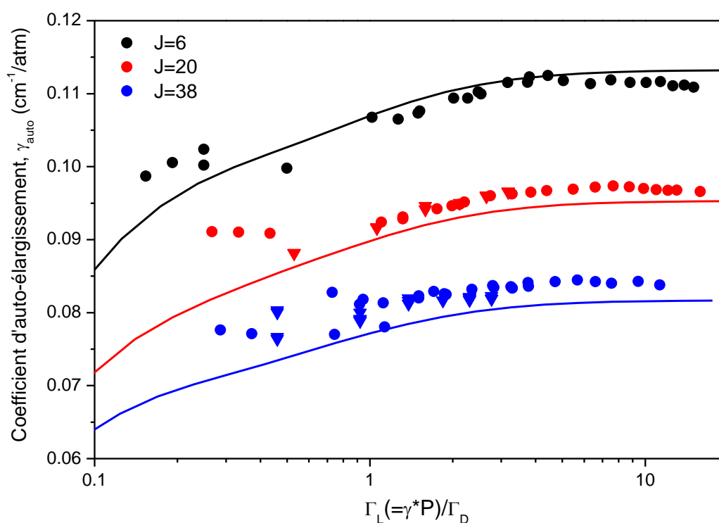
FIG. 7.7. Coefficient d'auto-élargissement obtenu par les ajustements par le VP des spectres observés (points) et calculés (lignes) en fonction du rapport \Gamma_L/\Gamma_D . Les \bullet sont les résultats obtenus par nos mesures dans la région de 1,6 \mu\text{m} et les \blacktriangledown sont ceux obtenus pour les mesures CRDS dans la région de 0,8 \mu\text{m} [Larcher 2014].
