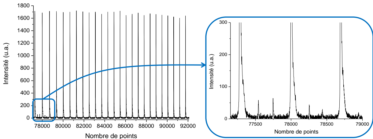
FIG. 3.10. Observation des pics d'interférences d'un mode parasite.
