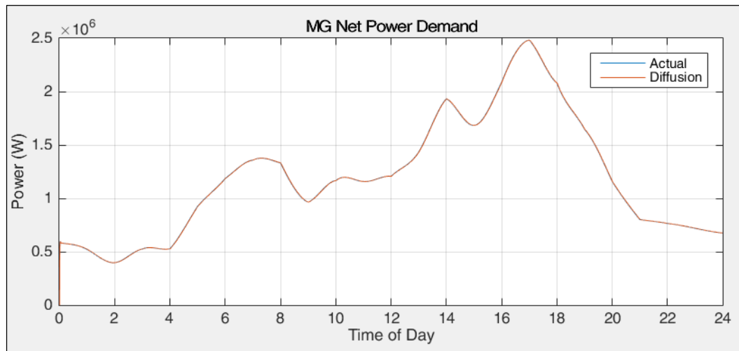
Figure 6.5.1: MG Net Power Demand, Actual vs Diffusion
