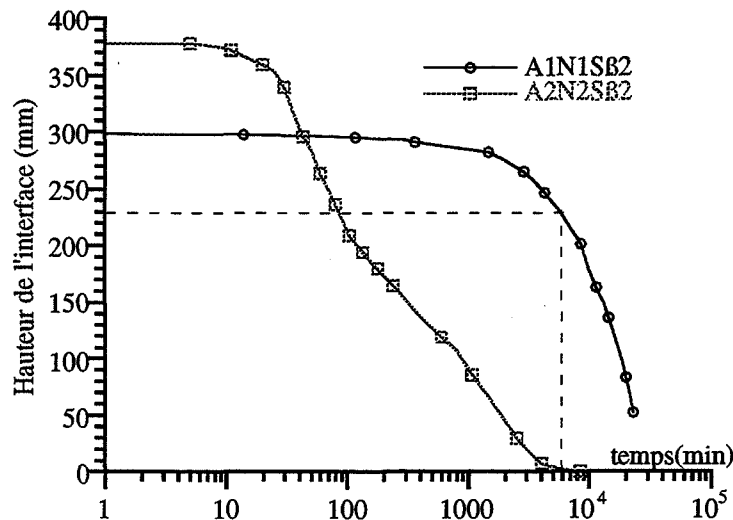
Fig. V.7 Chute de l'interface suspension-solvant, pour deux suspensions \text{A1N1S}\beta 1 et \text{A2N2S}\beta 2 .
