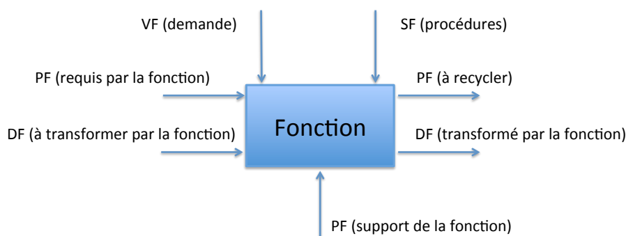
Figure 60 : Définition générique d'une fonction et de ses flux
