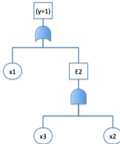
Figure 55 : Arbres de défaillance du système de distribution de fluide.
