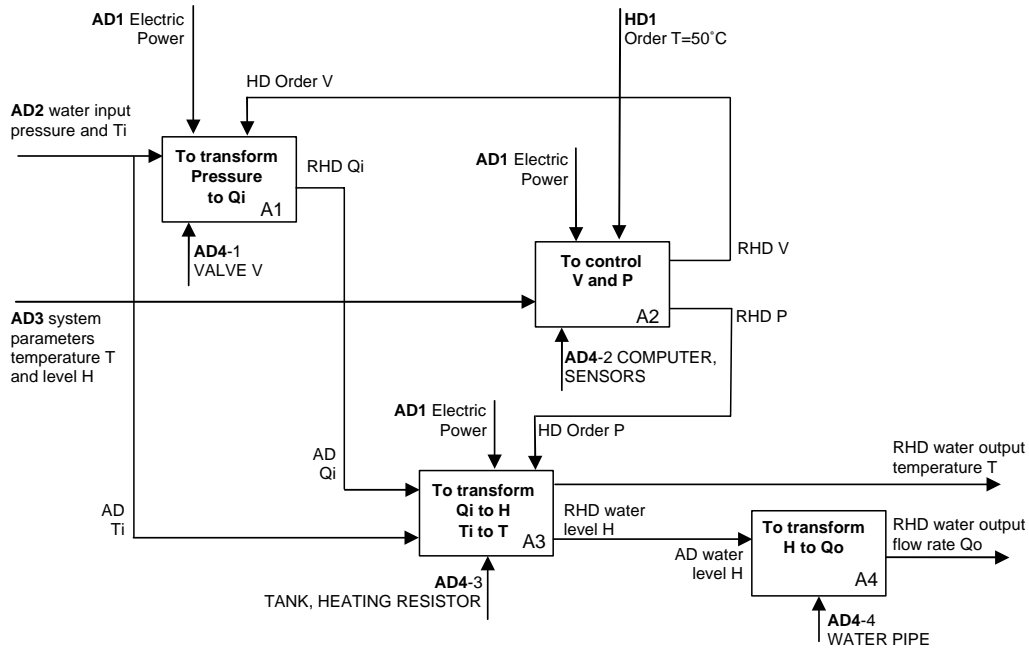
Fig. 25. SADT level A0.
