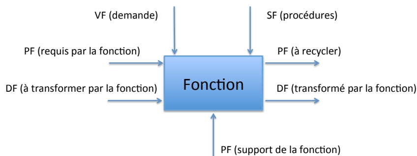
Figure 22 : Définition générale d'une fonction et de ses flux
