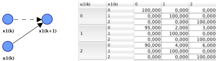
Figure 32 : Modèle RB Dynamique d'un MSM
