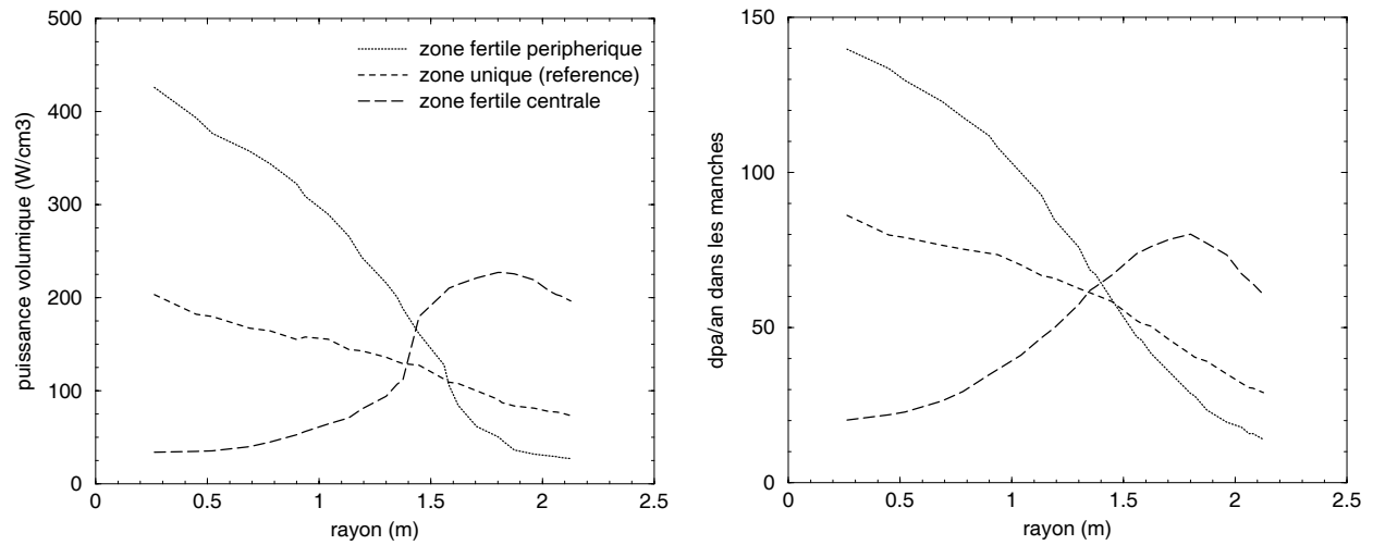
FIG. 5.3 – Répartition radiale de la puissance volumique et du taux de dommages dans le graphite selon la configuration du cœur.
