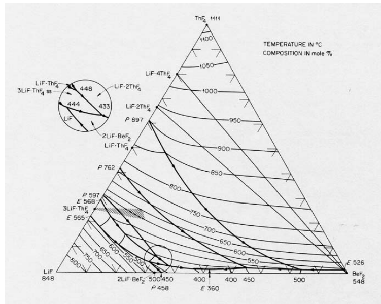
FIG. 2.6 – Diagramme de phase du sel LiF- \text{BeF}_2 - \text{ThF}_4 [29].
