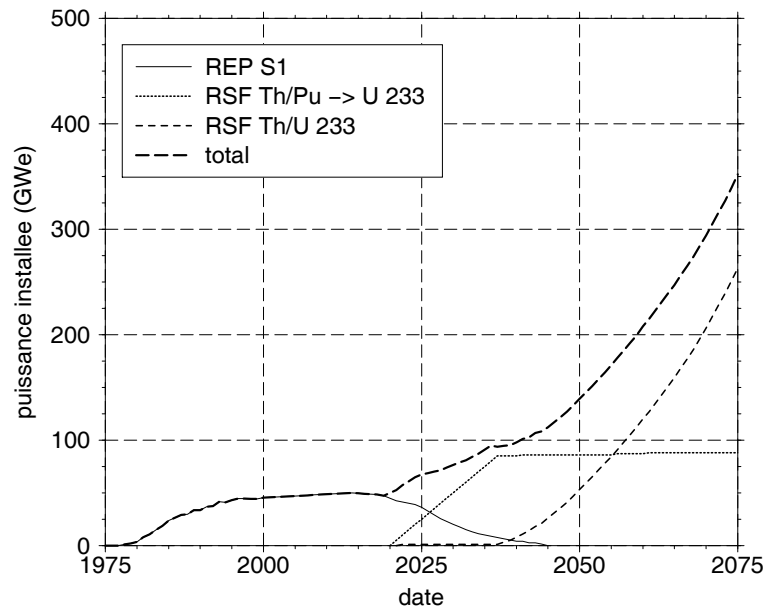
FIG. 6.38 – Scénario de déploiement basé sur l'utilisation optimale du plutonium des REP en RSF Th/Pu → ^{233}\text{U} et sur le démarrage de RSF ^{232}\text{Th}/^{233}\text{U} de référence, surgénérateurs.
