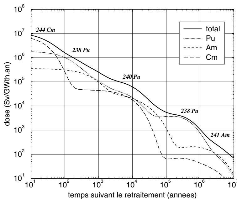
FIG. 6.6 – Evolution de la radiotoxicité des actinides rejetés 5 ans après le démarrage du RSF Th/Pu UOX 5 \rightarrow {}^{233}\text{U} . Les noyaux pères dont la radiotoxicité domine sont indiqués.
