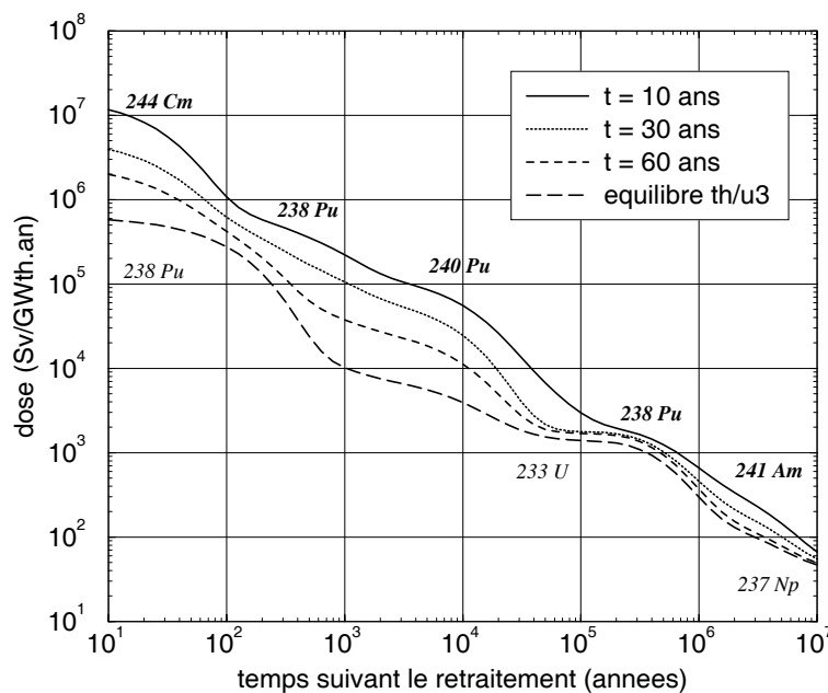
FIG. 6.7 – Radiotoxicité des actinides rejetés à différents instants t après le démarrage du RSF Th/Pu UOX 5 \rightarrow {}^{233}\text{U} , comparée à celle de l'équilibre {}^{232}\text{Th}/{}^{233}\text{U} (Les noyaux dominants dans ce cas sont indiqués sous la courbe correspondante en cas de changement).
