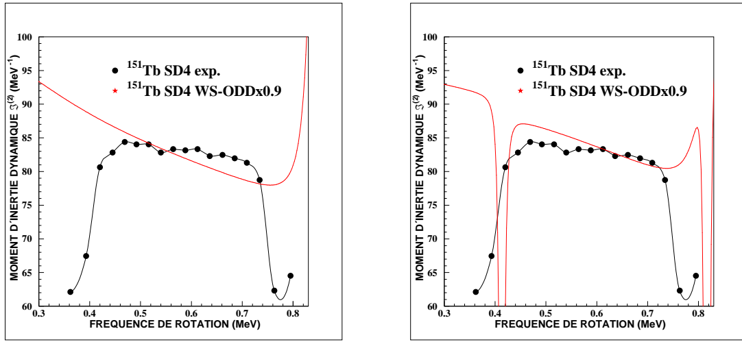
FIG. 4.14 – Moments d'inertie dynamiques de la bande superdéformée 4 du noyau ^{151}\text{Tb} . Les points noirs représentent les valeurs expérimentales et le trait rouge les valeurs calculées par un champ moyen avec un potentiel Woods-Saxon déformé et corrigées d'un facteur 0.9 pour reproduire l'effet du "pairing".
