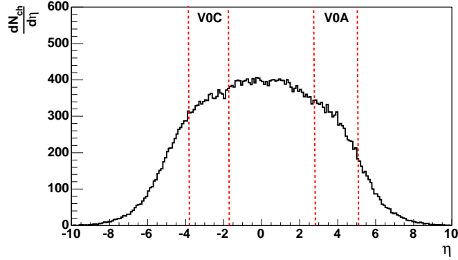
FIG. 4.11: Distribution en pseudo-rapidité des particules chargées produites dans des collisions Pb-Pb centrales ( 0 < b < 5 fm) à \sqrt{s} = 5.5 TeV. L'intervalle en pseudo-rapidité couvert par le V0A et V0C est indiqué par des traits pointillés.
