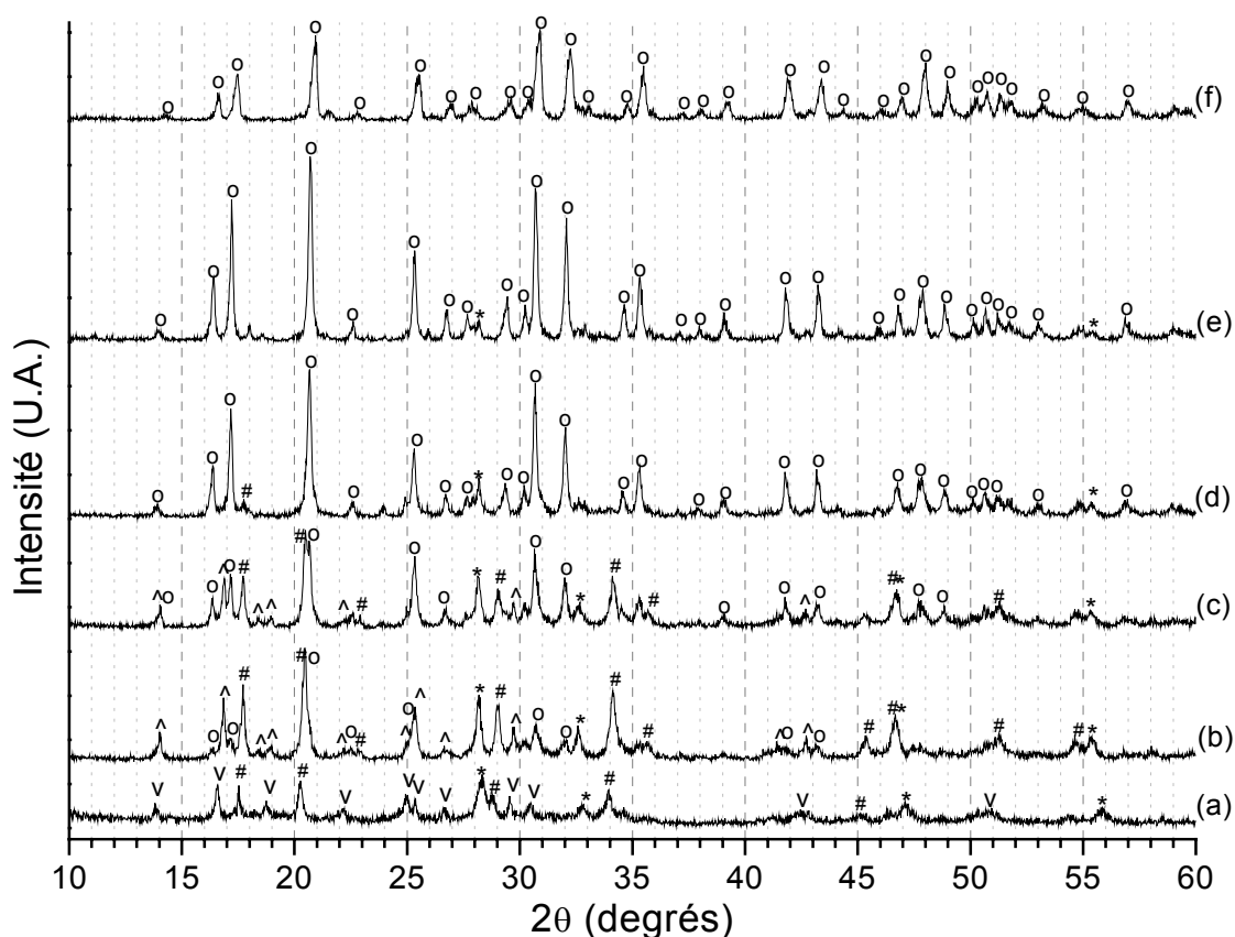
Figure 78. Diagrammes DRX enregistrés lors de la calcination d'un mélange de PHPTH, de UO_2 et de \alpha-ThP_2O_7 en fonction de la température de traitement thermique : \theta = 25^\circ C (a), \theta = 800^\circ C (b), \theta = 850^\circ C (c), \theta = 900^\circ C (d), \theta = 1000^\circ C (e) et \theta = 1150^\circ C (f). Raies caractéristiques du PHPTH (v), de \alpha-ThP_2O_7 (#), de UO_2 (*), de \alpha -PDT (^) et du \beta -PDTU (o).
