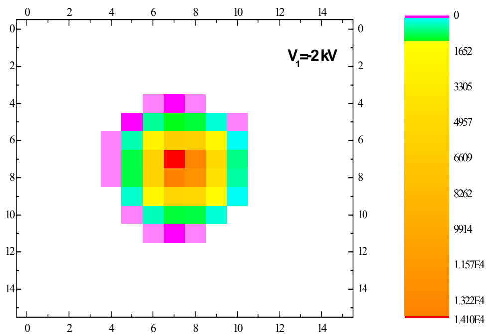
Figure 13 Image bidimensionnelle de (CsI)I émis à l'impact de Au_9^+ de 50 keV/atome. V_1 = -2kV
