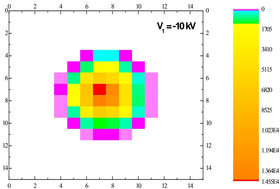
Figure 14 Image bidimensionnelle de (CsI)I émis à l'impact de Au_9^+ de 50 keV/atome. V_1 = -10kV
