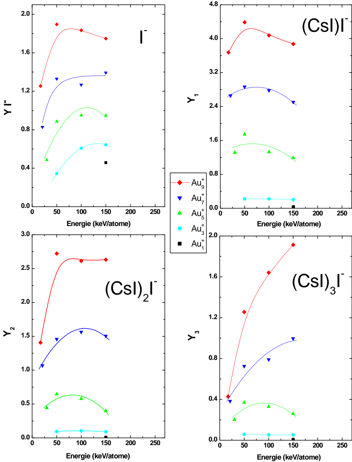
Figure 11 : Rendements d'émission de \Gamma , (CsI)\Gamma , (CsI)_2\Gamma et de (CsI)_3\Gamma mesurés avec le détecteur multi-anode LAG en fonction de l'énergie par atome des agrégats Au_n^+ .
