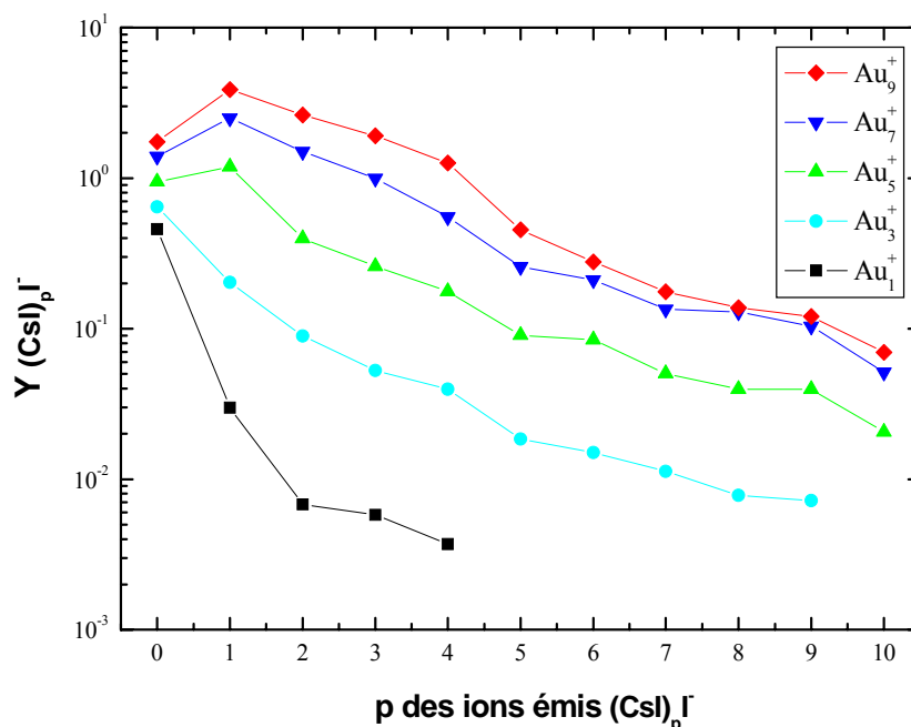
Figure 7 : Rendements d'émission des ions (\text{CsI})_p\text{I}^- en fonction de leur taille p , mesurés avec le détecteur multi-anode à l'impact des projectiles \text{Au}_n^+ ( n=1 à 9 ) de 150 keV/atome.
