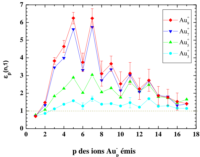
Figure 5 : Variation du facteur de non linéarité ε p (n,1) en fonction de la taille p des agrégats Au p + émis à l'impact des différents agrégats Au n + incidents.
