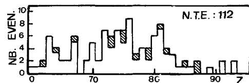
FIG. 4. — Distribution des 112 événements du rayonnement cosmique observés à bord de Skylab d'après [15] les zones hachurées indiquent des résultats pouvant être éventuellement révisés.
