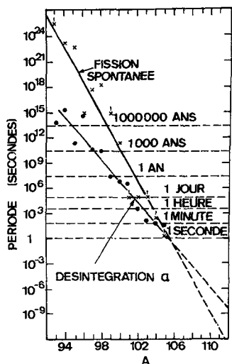
FIG. 1. — Durées de vie les plus longues des éléments transuraniens connus (d'après G. T. Seaborg [18]).
