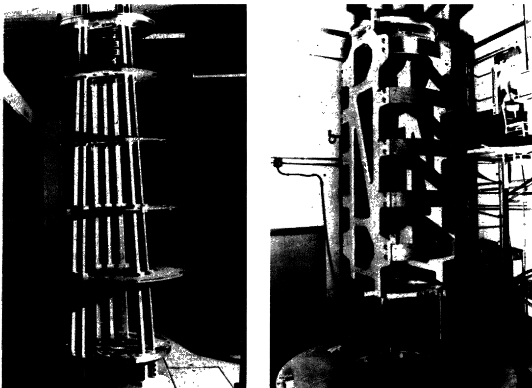
Fig. 8. — Différentes phases des essais et tests réalisés au CRN sur les isolants et sur une section du générateur haute tension. [Different steps of the tests performed at the CRN on insulators and on one section of the high voltage generator.]
