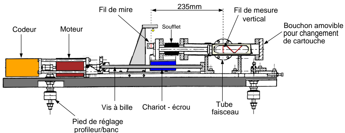
Figure 2.3 - Coupe transversale du profileur à fil adopté pour le projet ARC ("ARC Scanner"). L'équipage mobile est représenté en position de référence : le fil de mesure vertical est sur l'axe du faisceau nominal.
