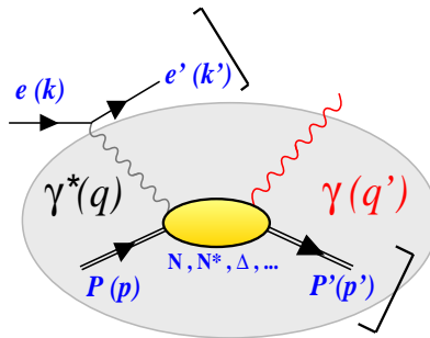
Figure 1.5 - Réaction de photo-électroproduction sur le proton. Le processus de diffusion Compton virtuelle qui nous intéresse est représenté en grisé. Dans cette réaction, le photon virtuel \gamma^* est échangé entre l'électron et le proton. L'état intermédiaire ainsi formé décroît en rayonnant un photon réel. Expérimentalement, on détecte en coïncidence l'électron et le proton diffusé.
