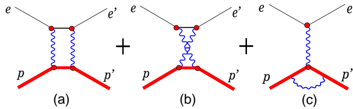
Figure 2.5 - Graphes (a) et (b) : graphes mettant en jeu l'échange de deux photons virtuels entre les bras hadronique et leptonique. Graphe (c) : correction de vertex sur le proton.
