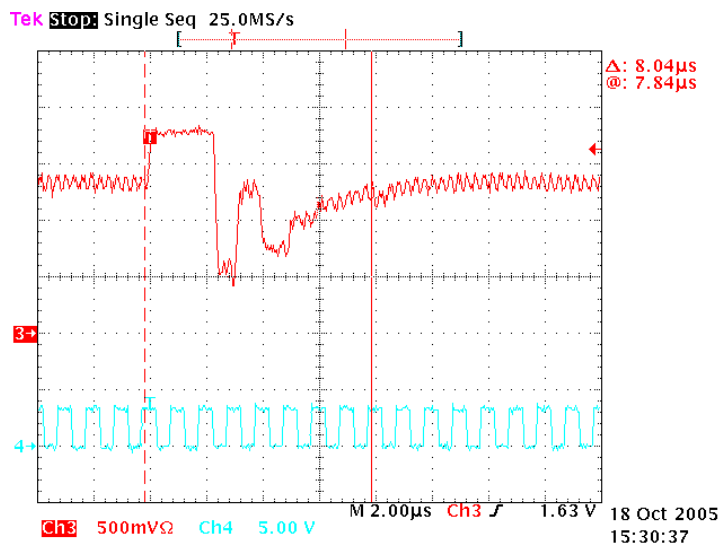
Figure 3-5 : Compensation d'offset : la variation de la ligne de base suit la sortie du comparateur, en rouge la sortie du buffer (Buf_ampli10), en bleu l'entrée d'horloge (Clk).
