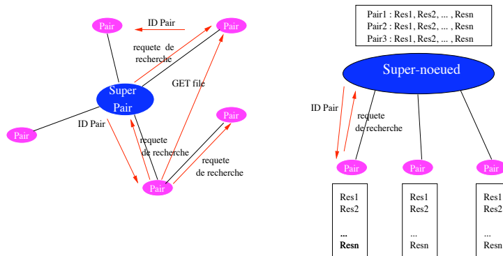
FIG. 2. A gauche un super-Pair du système Clip2 et à droite un super-noeud du système FastTrack.
