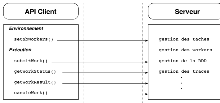
FIG. 6. Fonctions de l’API Client
