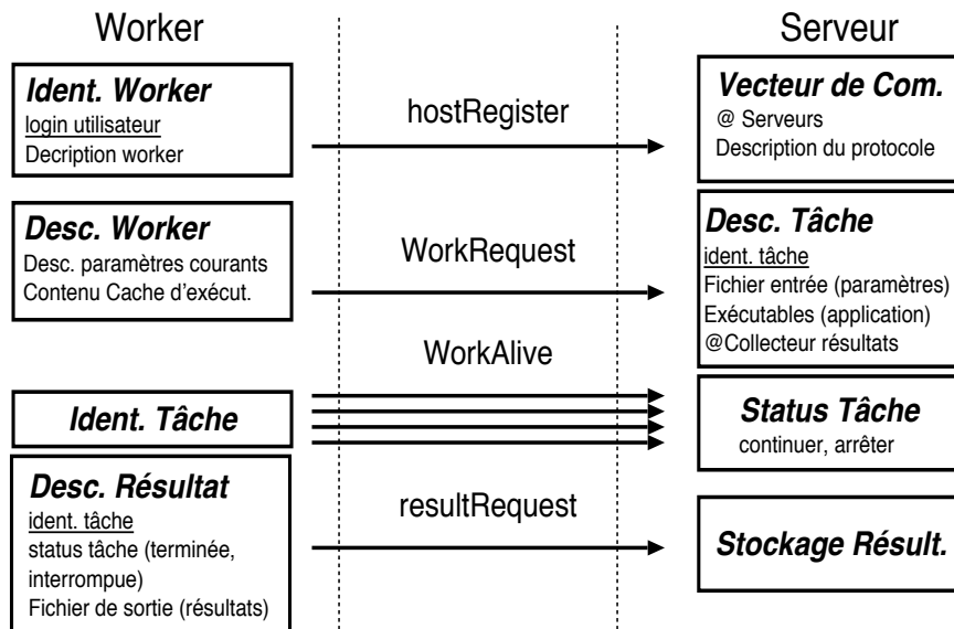
FIG. 5. Le protocole entre le serveur et un Worker
