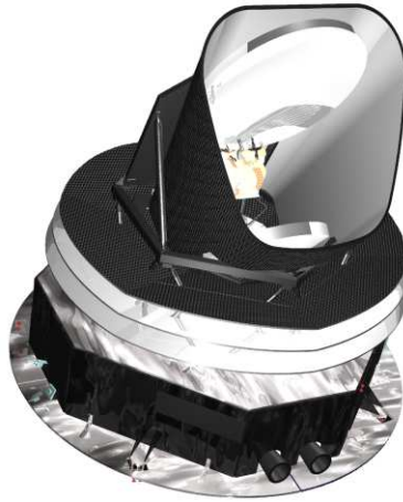
FIG. 5.1 – Vue d’artiste du satellite PLANCK. Nous pouvons distinguer le télescope avec ses miroirs primaire et secondaire illuminant le plan focal, l’enceinte de protection du télescope, les cônes d’isolation thermique ainsi que le panneau solaire.
