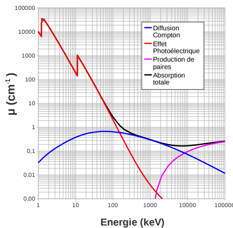
FIGURE A.4 – Coefficient linéique d'atténuation \mu dans le germanium.
