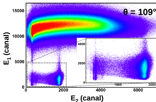
FIGURE 4.21 – Matrice N(E_1, E_2) brute pour le télescope à 109^\circ .
