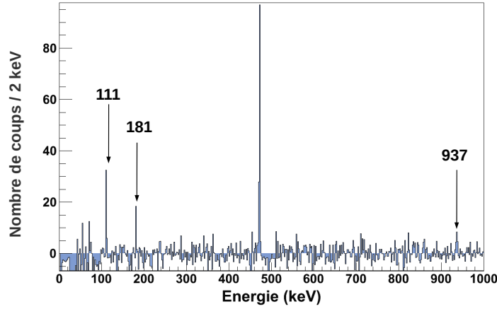
FIGURE 5.20 – Spectre \gamma en coïncidence avec la raie à 1692 keV.
