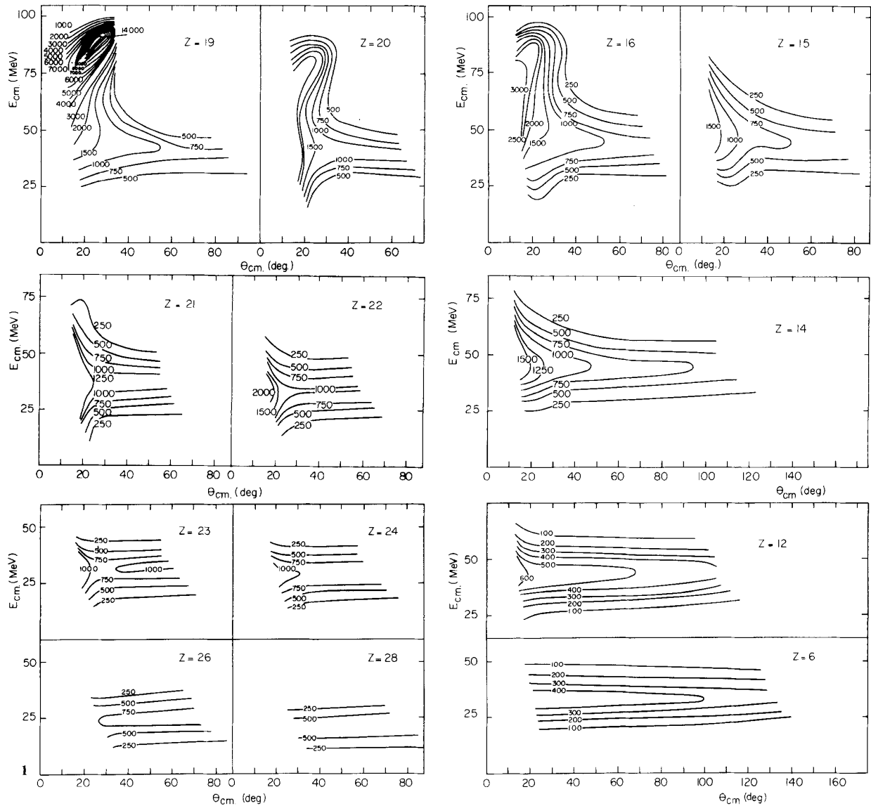
FIGURE 3.14 – Diagrammes de Wilczynski obtenus pour différentes valeurs du nombre de protons dans la réaction ^{40}\text{Ar} (280 \text{ MeV}) + ^{58}\text{Ni} [Gatt 75a]. La section efficace (d^2\sigma/(dE \cdot d\theta))_{CM} est donnée en \mu\text{b}/(\text{MeV} \cdot \text{rad}) .
