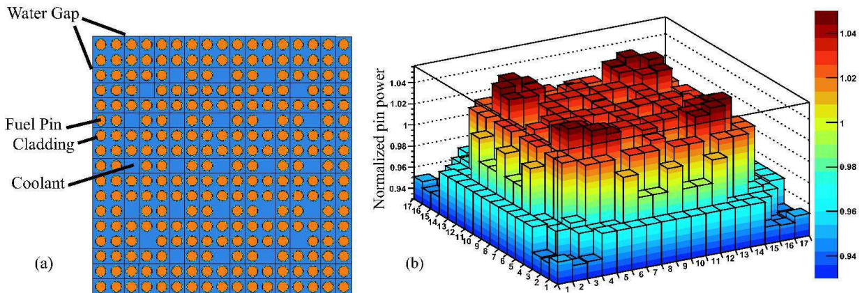
FIG. 2.7 – Modèle d'assemblage REP-N4 (a) et distribution de puissance par crayon (normalisée à la puissance moyenne) pour un tel assemblage UOX en début de cycle (b).
