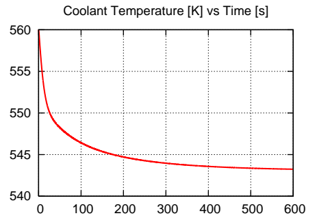
FIG. 5.5 – Jeu initial des paramètres thermiques ou cinétiques (a) et résultats (b) calculés par CheckPoint pour le transitoire "UTOP min" du CANDU ^{nat}\text{U} (BOC) avec \Delta\rho_{min} = -390 pcm.
