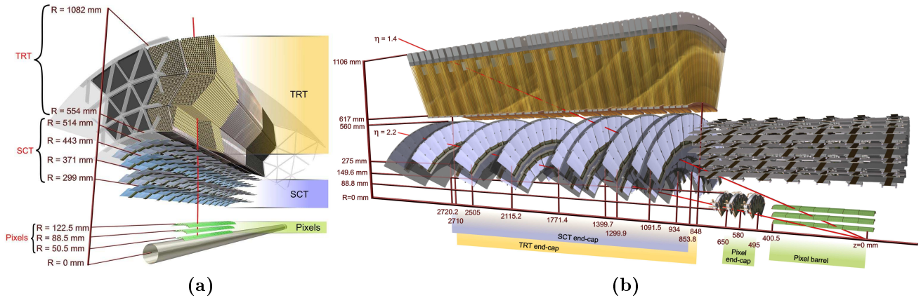
Figure 3.5 : Composants du détecteur interne d'ATLAS dans la partie tonneau (a) et un des bouchons (b).
