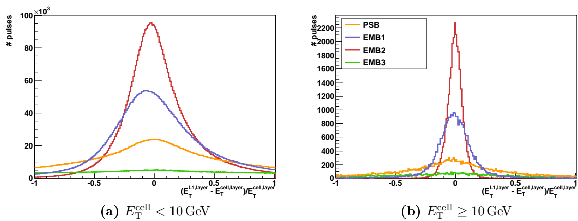
Figure A.15 : Distributions des erreurs relatives sur les énergies dans différentes couches, estimées à partir des énergies du L1Calo calibrées, pour E_T^{cell} < 10 GeV (a) et E_T^{cell} \geq 10 GeV (b).
