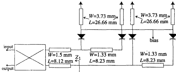
Fig. 2. Phase shifter
