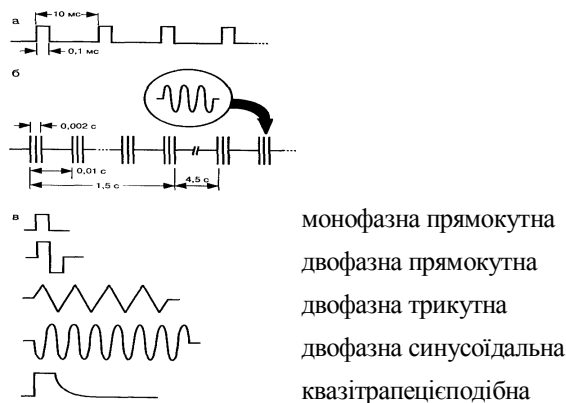
Рис. 5.8. Вибрані режими стимулів, що використовуються у процесі нервово-м'язового стимулювання: а) умовний ряд низькочастотних (100 Гц) стимулів з шириною імпульсу 0,1 мс; б) структура високочастотного стимулювання (10 кГц, синусоїдальна хвиля), що моделюється при низькій частоті (100 Гц) з інтервалом між послідовними стимулами 0,01 с; в) форма хвиль, що використовуються у процесі нервово-м'язового стимулювання; двофазні форми хвиль коливаються відносно нульової лінії
