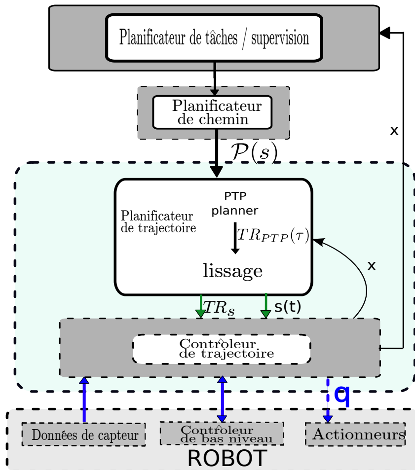
Figure C.2: Le contrôleur de trajectoire se trouve à un niveau intermédiaire de l'architecture du contrôleur, entre les contrôleurs rapides des axes du robots et le niveau planification plus lent.
